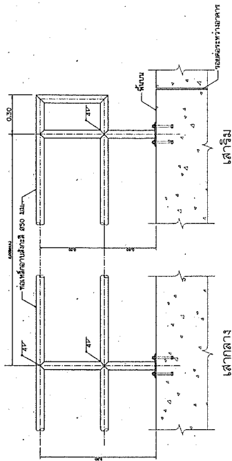
รูปด้านข้างเสาเข็ม ไม่แสดงขนาด
