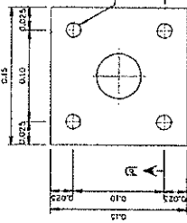
รูปขยายแผนหลักหน้าแปลน
