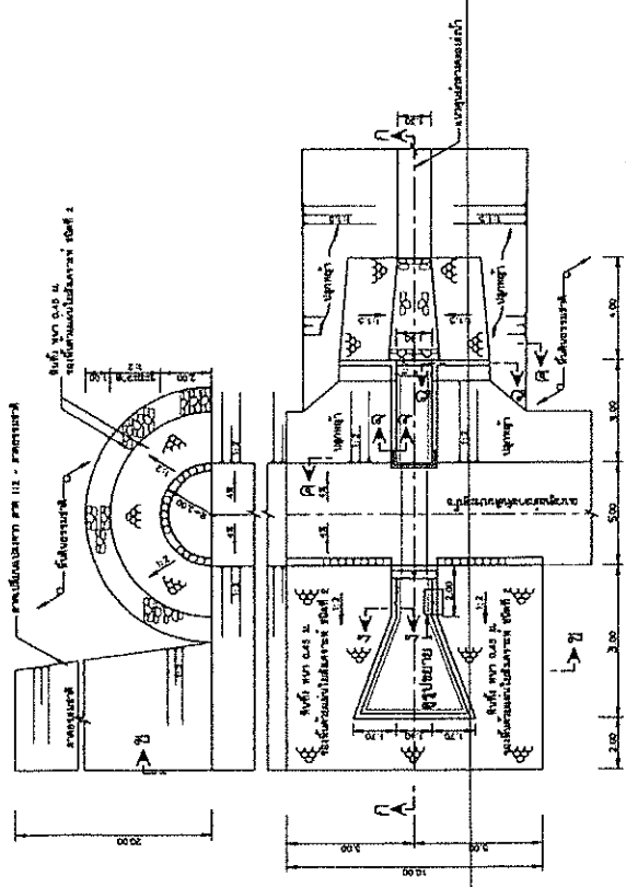
แปลนอาคารบังคับน้ำแบบผ่าท่อสำหรับฝายน้ำล้น
