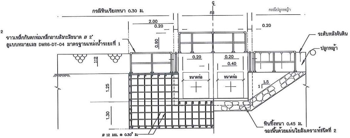
รูปตัด ง-ง มาตราส่วน 1:50
