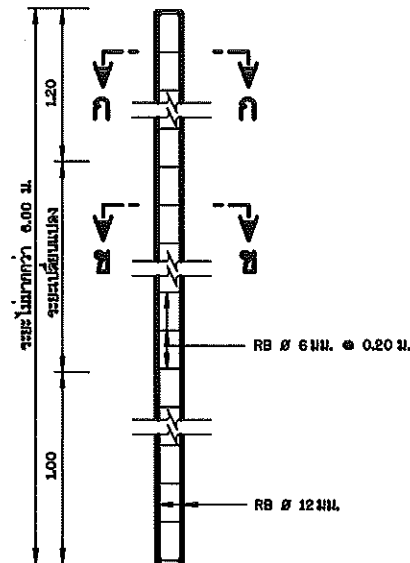
รายละเอียดเข้าป้าย คสล.
