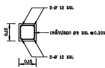
รูปตัด ก - ก
