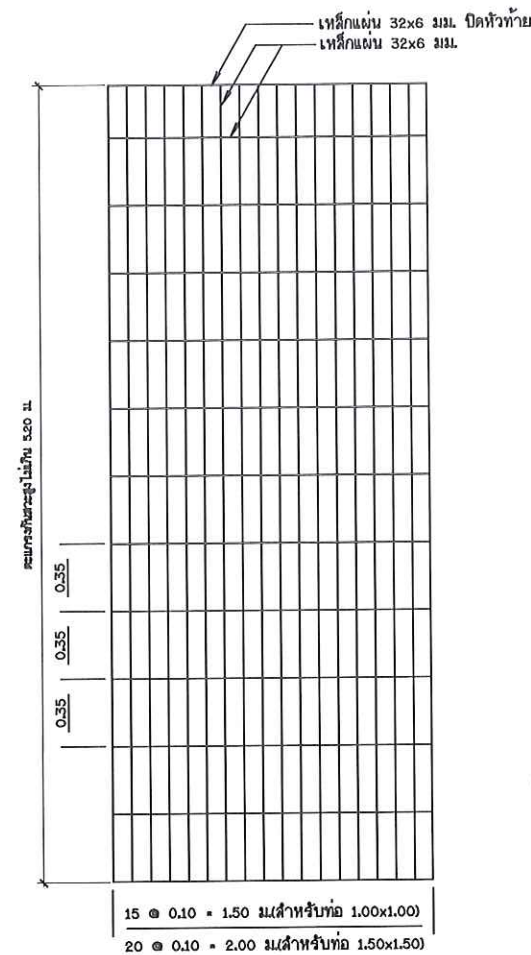
แบบขยายตะแกรงกันสวะ
