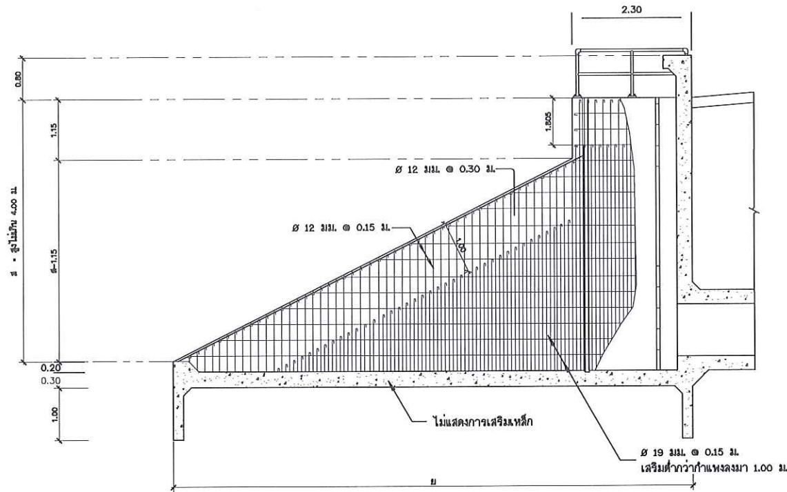
แสดงการเสริมเหล็กกำแพงด้านข้างอาคารเหนือฝ้า ไม่แสดงขนาดราส่วน
