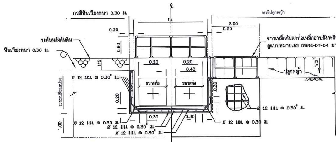
รูปตัด ค-ค มาตราส่วน 1:50
