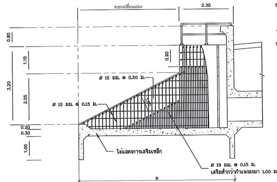
ตัวอย่างแสดงการเสริมเหล็กกำแพงด้านข้างอาคารเหนือฝ้า
