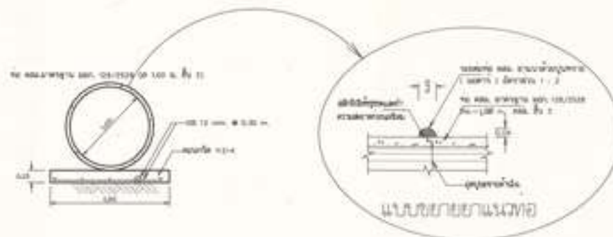
รูปตัด 2-2 (ขนาด 1.00 ม.) ขนาด 1:100
