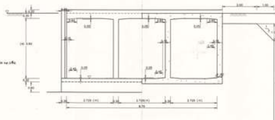
รูปตัด C - C
