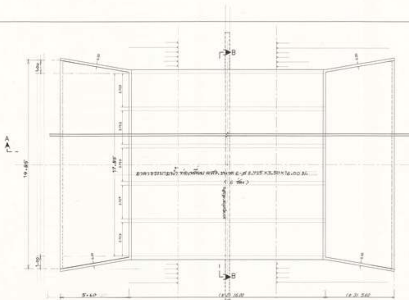
แปลนอาคารระแนงน้ำ มาตราส่วน 1:75
