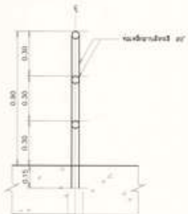
รูปตัด A - A ขนาดส่วน 1:25
