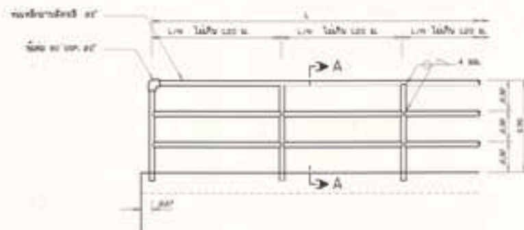
รูปขยายราวเหล็กกันตก ขนาดส่วน 1:25
