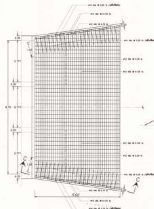
แสดงการเสริมเหล็กปากท่อน คสล.
