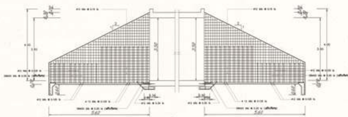
รูปตัดขยายการเสริมเหล็กแนว C - C ขนาด 1:50
