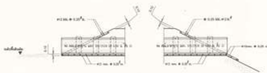
รูปขยาย ① ขนาด 1:20
