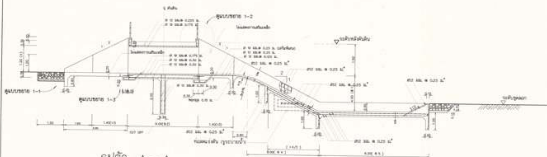
รูปตัด A - A มาตราส่วน 1:500
