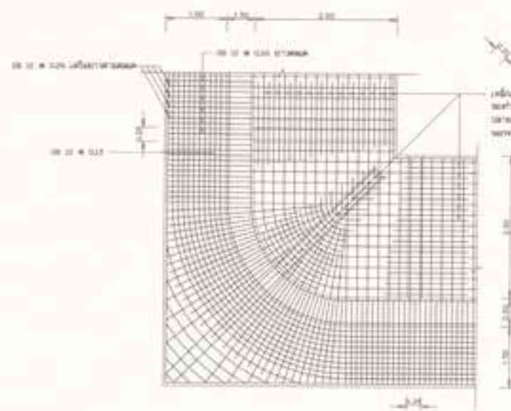
แผนแสดงเหล็กเสริมด้านบน 1 : 50
