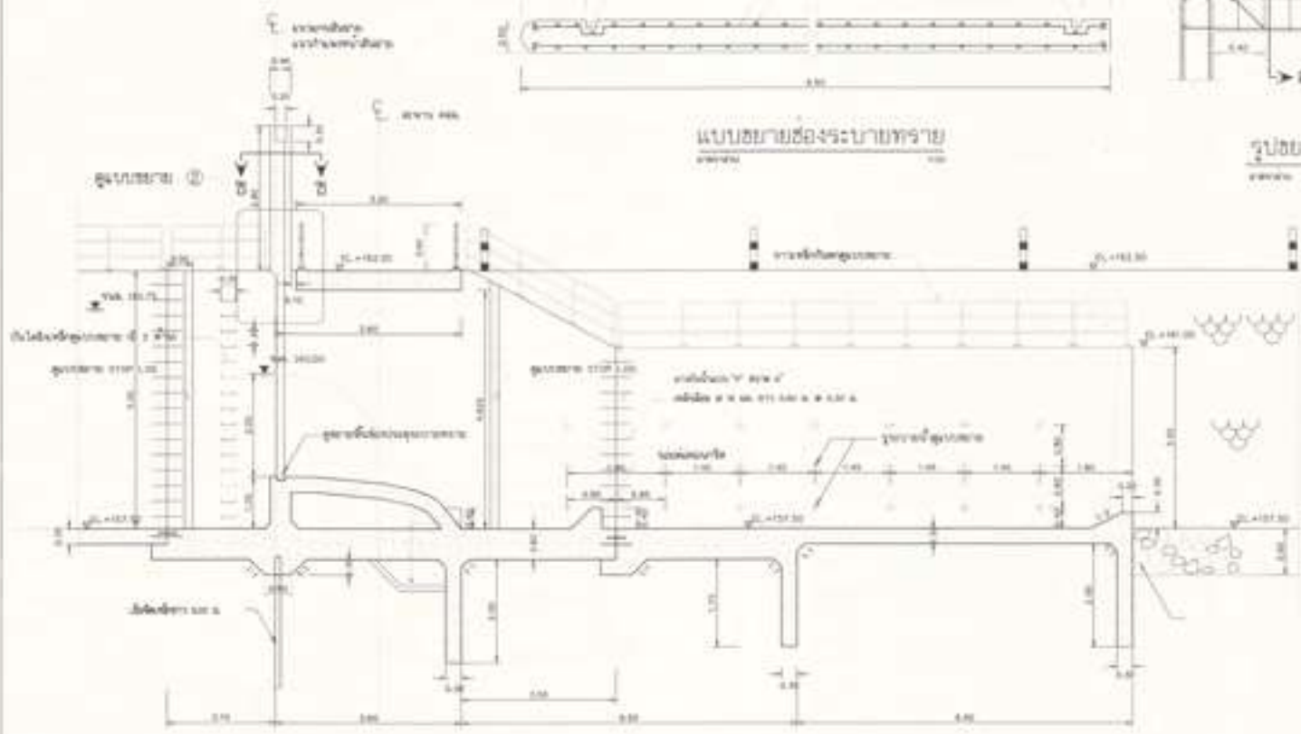
รูปตัดช่องระบายทรายตามแนว ก-ก
