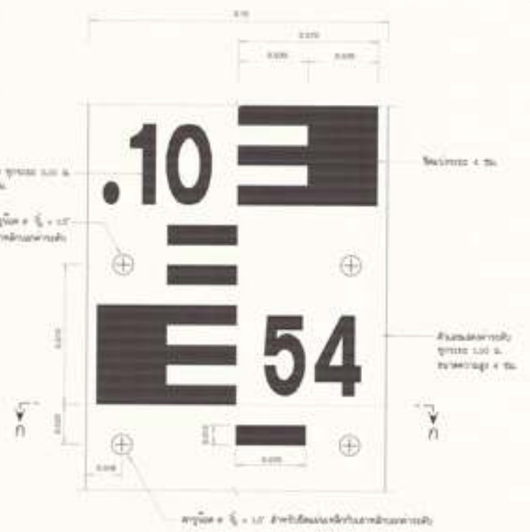
ขยายแผ่นเหล็กบอกค่าระดับ ขนาดจริง 1:1
