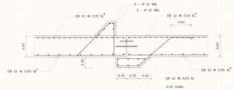
แสดงการเสริมเหล็กแบบขยาย 4-ก ขนาด 1:25
