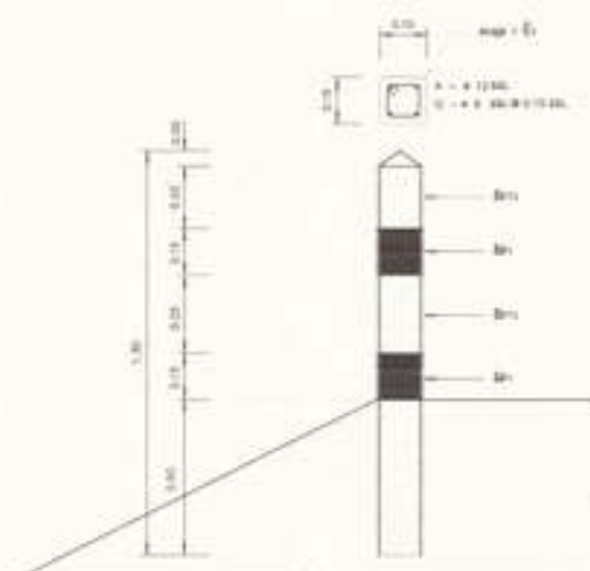
แบบขยายหลักริมคันดิน ขนาด 1:10
