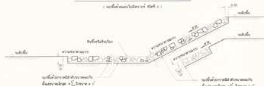
รูปตัดแสดงการเรียงหิน (แบบที่ 2)
