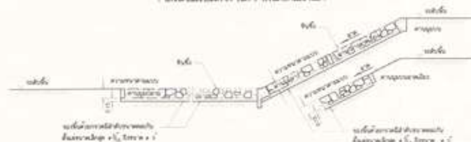
รูปตัดแสดงการเรียงหิน (แบบที่ ๔)
