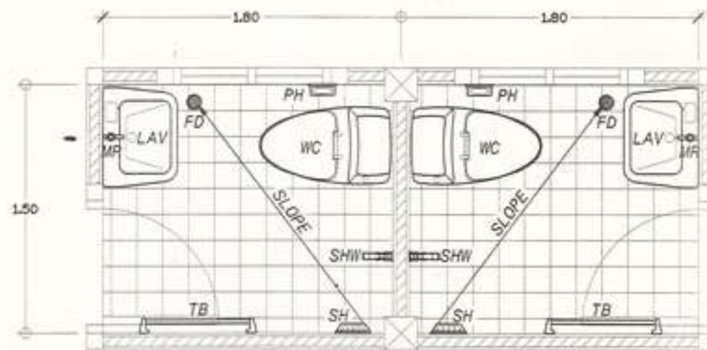
แบบขยายห้องน้ำ
