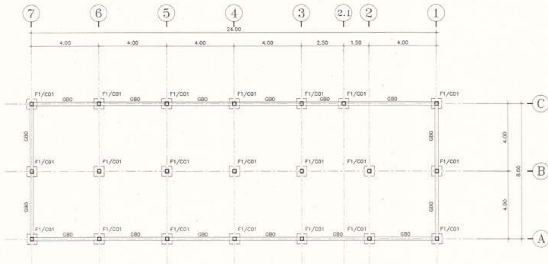
แปลนฐานราก/คานคอดิน ขนาดส่วน 1 : 100
