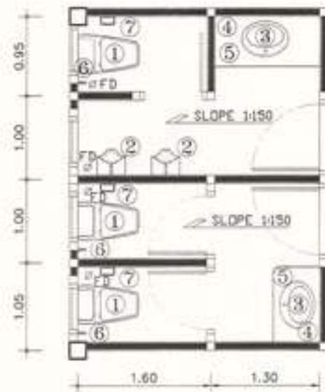
แบบขยายห้องน้ำ มาตราส่วน 1 : 30
