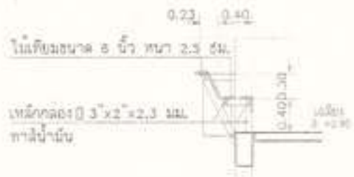
รูปตัด 1
