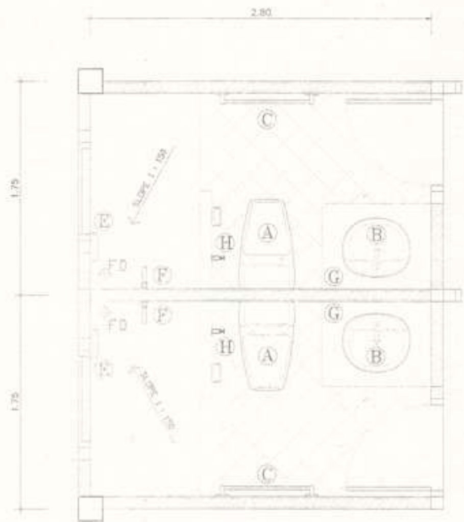
แบบขยายห้องน้ำ ขนาดพื้นที่ 10.00 ตร.ม. 1 : 25
