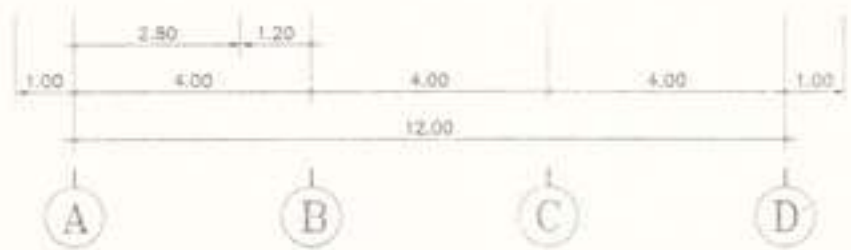
รูปด้านหน้า 1 : 100
