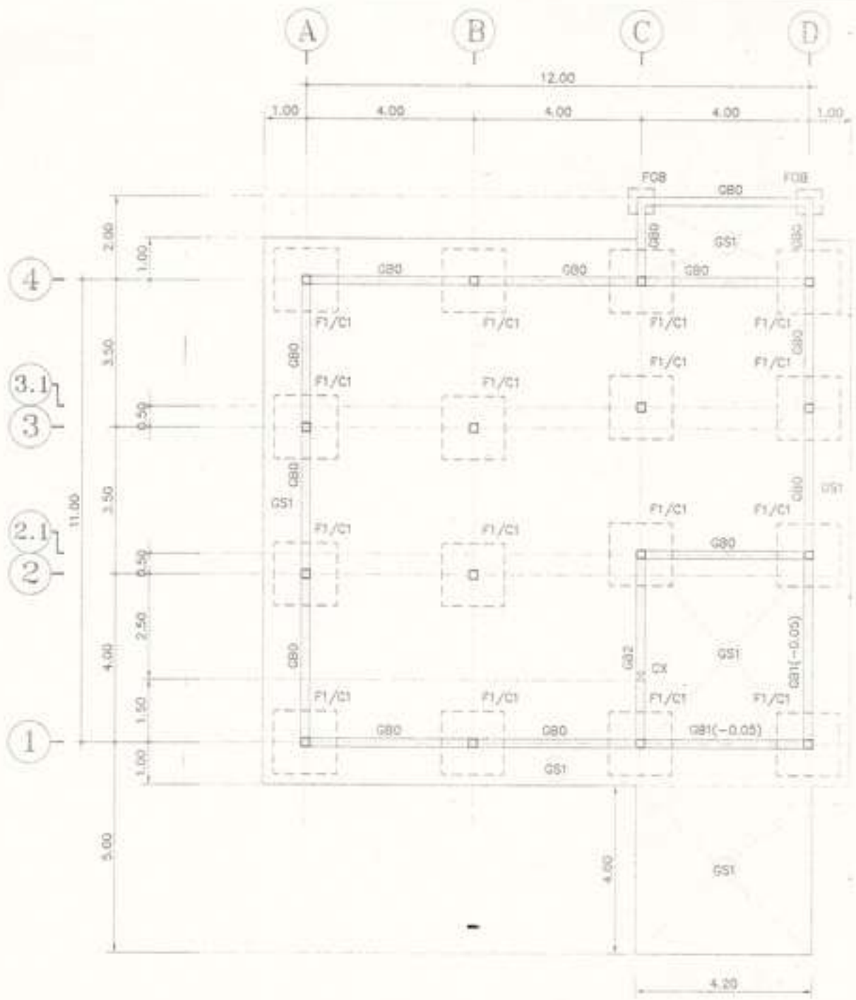
แปลนฐานราก/ตอม่อและคานคอดิน 1 : 100
