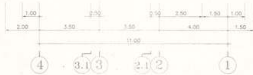
รูปด้านข้างซ้าย บ้านสวน 1 : 100
