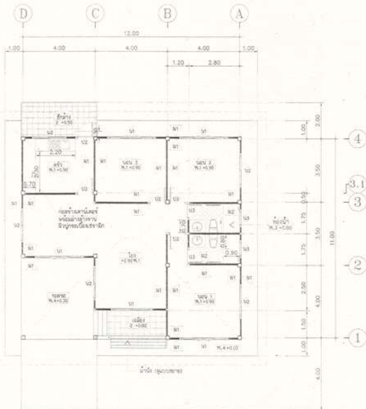
แปลนพื้น (แบบกลับ) ขนาดรวม 1 : 100
