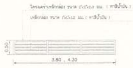
แบบขยายแผงกันแดด 1:50
