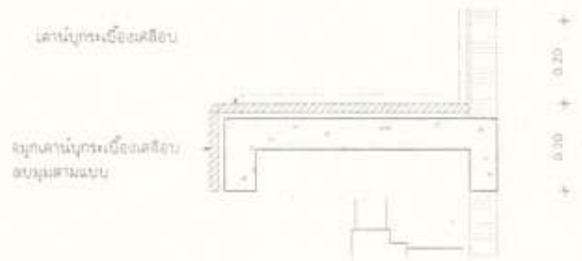
แบบขยายเคาน์เตอร์ หน้าตัด 1/18
