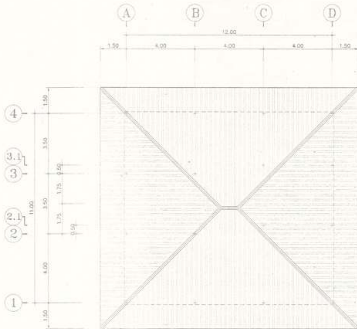
แปลนหลังคา ขนาดส่วน 1 : 100
