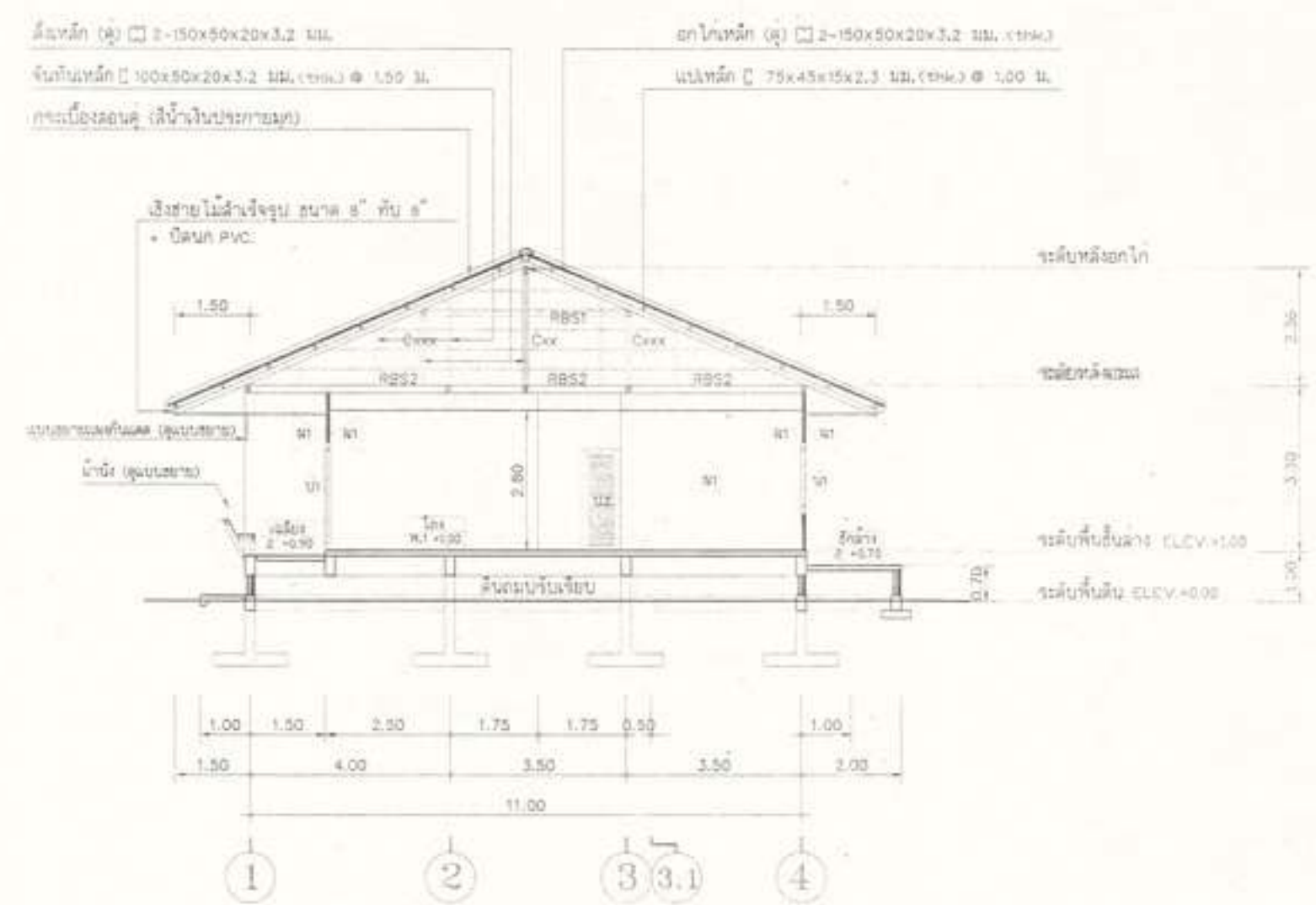
รูปตัด B-B อัตราส่วน 1:50
