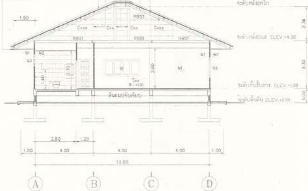
รูปตัด 1 : 100
