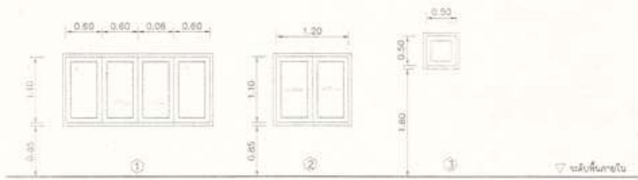
แบบขยายประตู-หน้าต่าง ขนาดจริง 1:50
