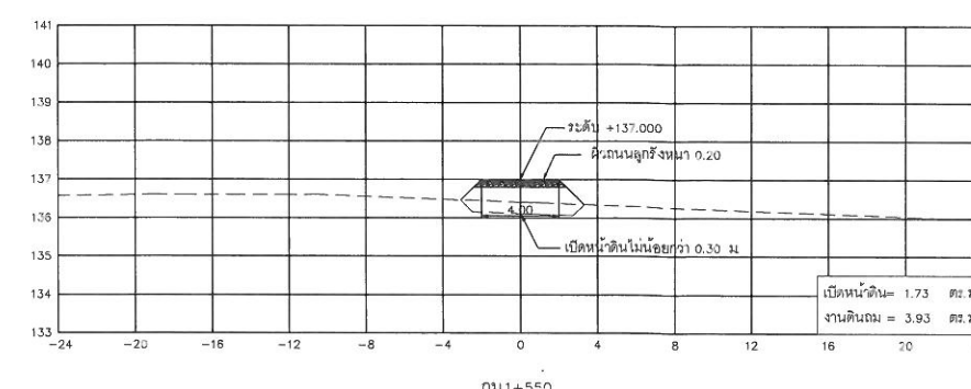
กม.1+550
