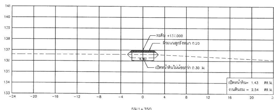
กม.1+350
