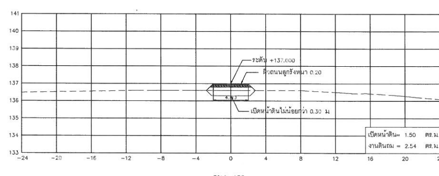
กม.1+450
