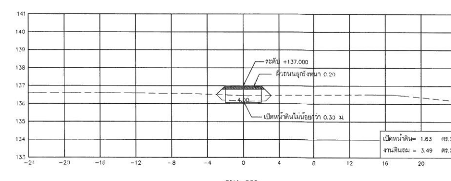
กม.1+500
