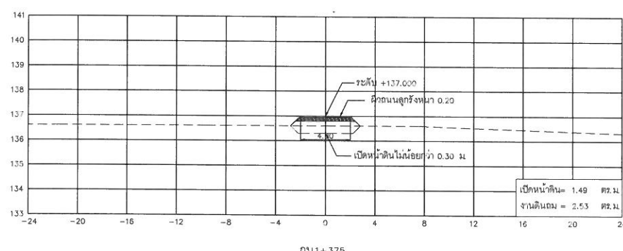
กม.1+375
