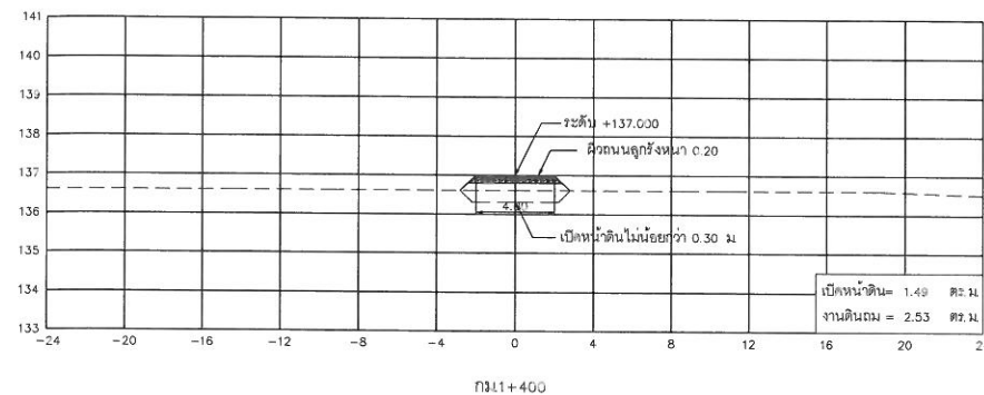
กม.1+400
