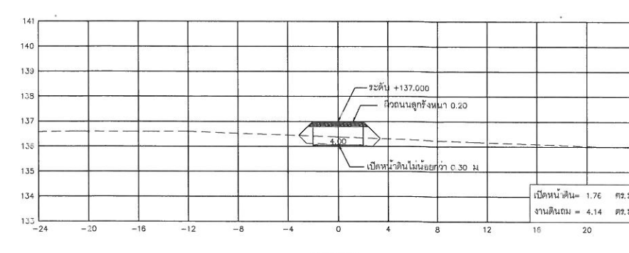
กม.1+525
