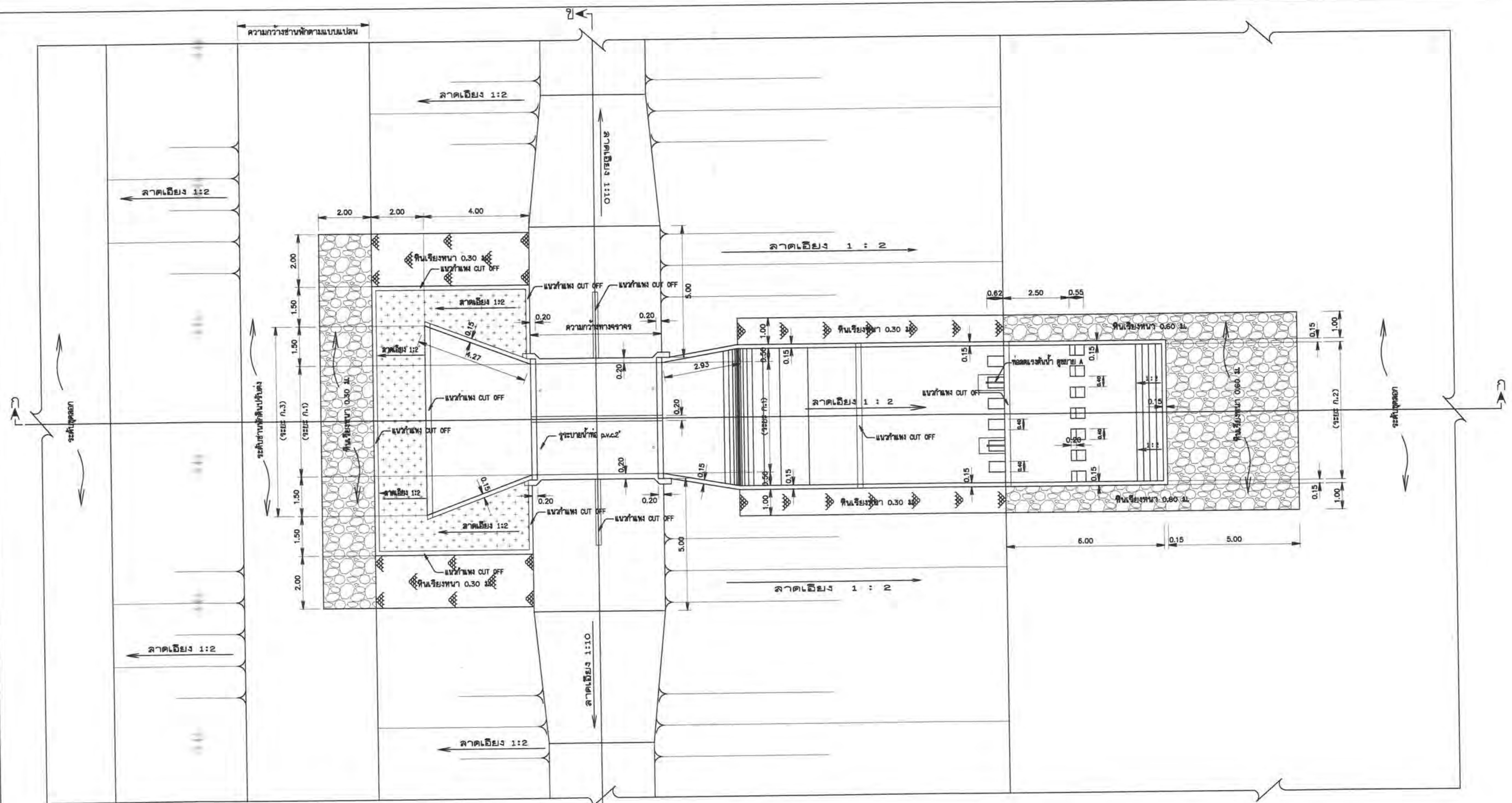
แปลนอาคารระบายน้ำ : ๕/๑
