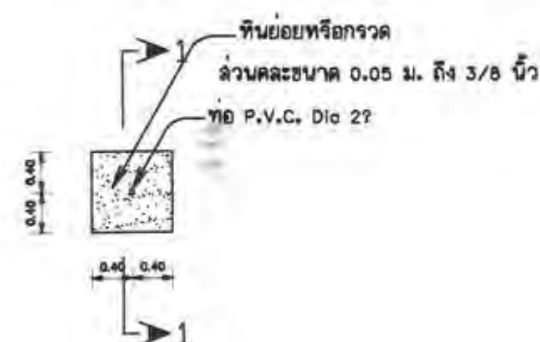
แปลนระบายน้ำของพื้น คสล. ลาดเอียง ขยาย A มาตราส่วน 1 : 50
