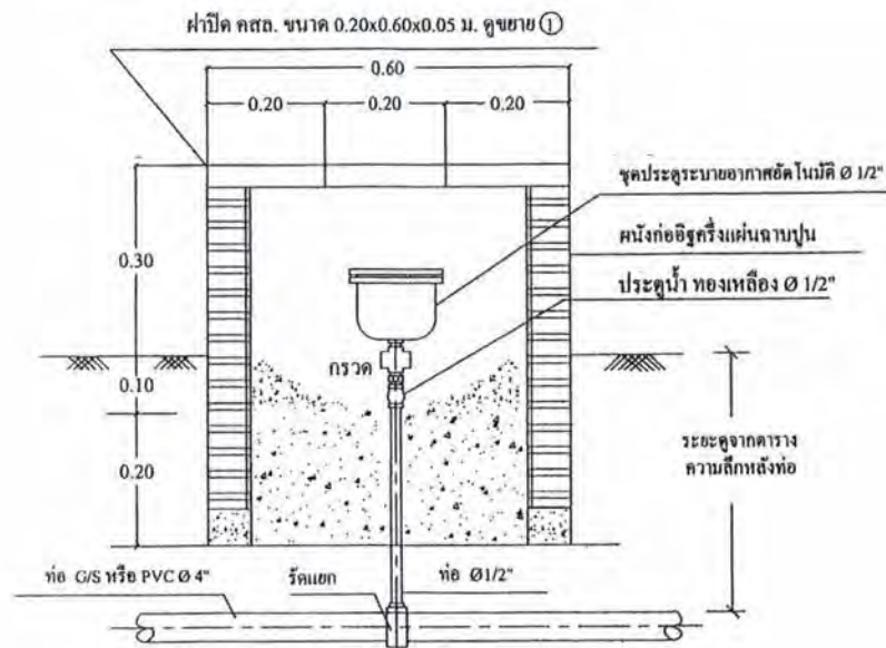
11. การติดตั้งประตูลมอากาศอัตโนมัติ
