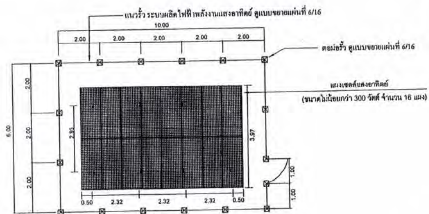
แปลนการติดตั้งแผงเซลล์แสงอาทิตย์ พร้อมมั่ว
