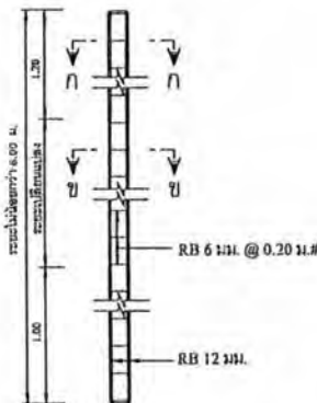
รายละเอียดเสาป้าย กสท. มาตราส่วน 1:20
