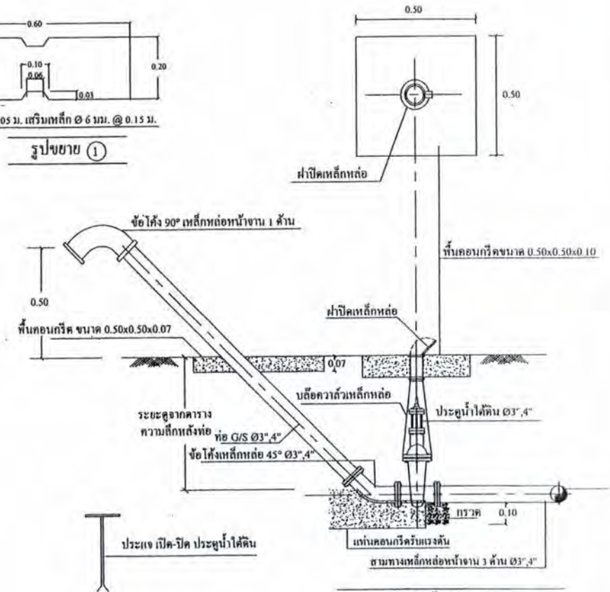
13. แบบการติดตั้งประตูลมอากาศอัตโนมัติ
