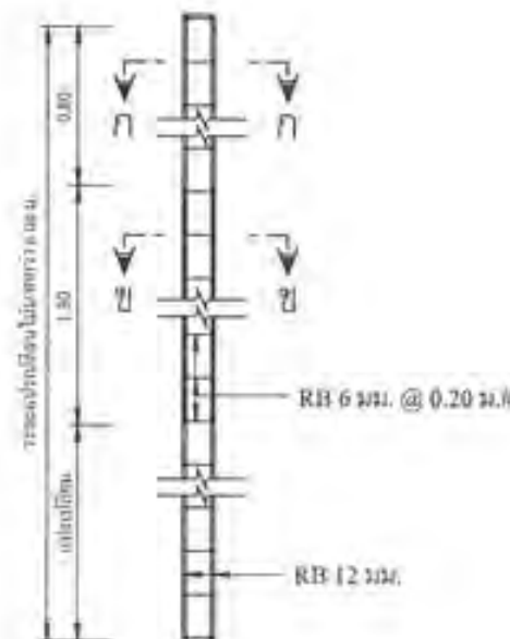
รายละเอียดเสาป้าย กสส.
