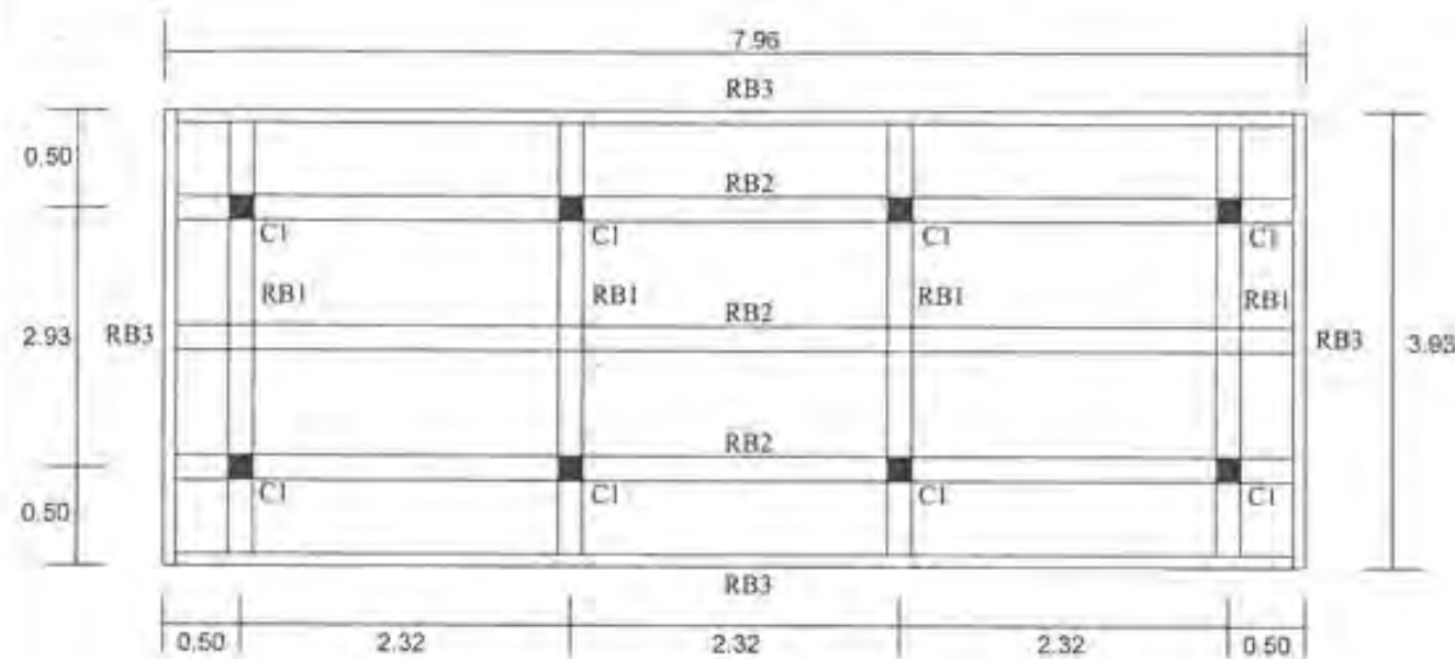
แปลนคานโครงสร้างคาน
