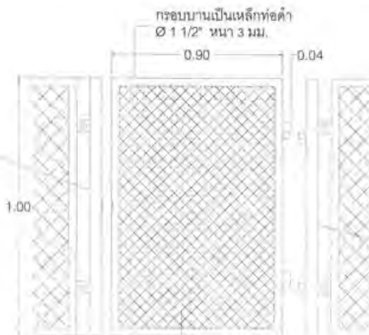
รูปตัด A แบบขยายรายละเอียดแสดงการยึดระหว่างรั้วกับเสา
