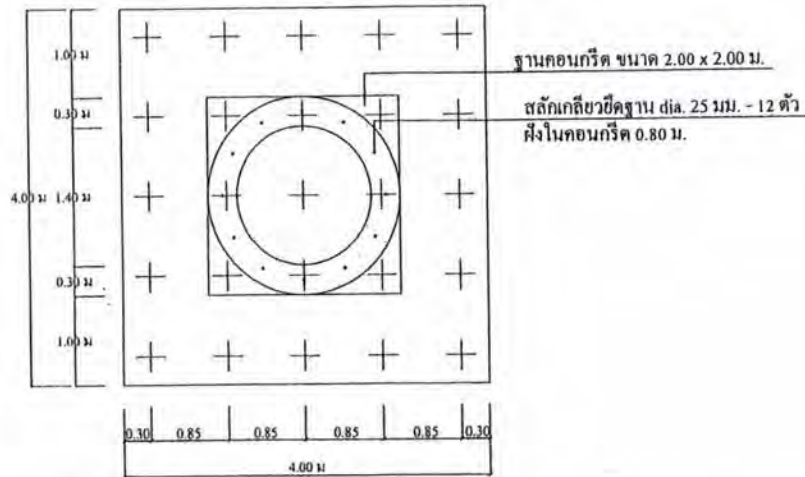
แบบขยายฐานรากหอดังสูง แบบมีเสาเข็มและไม่มีเสาเข็ม
