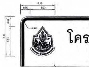
ป้ายโครงการ มาตราส่วน 1:20
