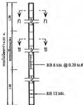
รายละเอียดภายใน กสท. มาตราส่วน 1:30
