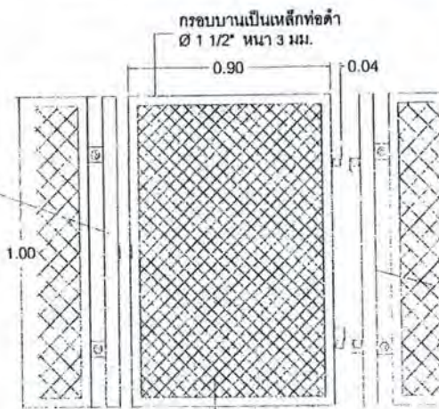
รูปตัด A แบบขยายรายละเอียดแสดงการยึดระหว่างรั้วกับเสา
