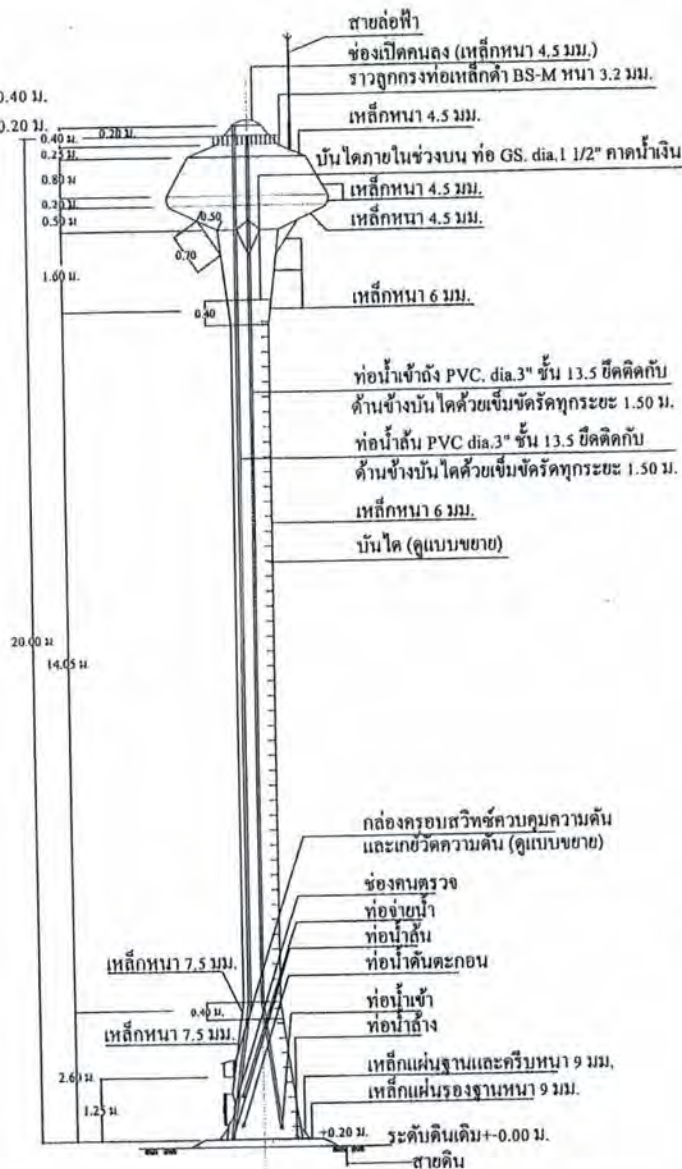
รูปด้านข้างของถังสูง แบบถังเหล็กรูปทรงแอมแปม มาตรฐาน 1 : 100
