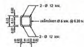
รูปตัด ข - จ
