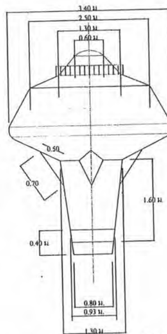
แบบขยายแมนโซลบนของถังสูง มาตรฐาน 1 : 50
