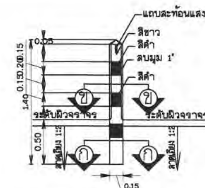
รูปขยายหลักบอกแนว มาตราส่วน 1:25
