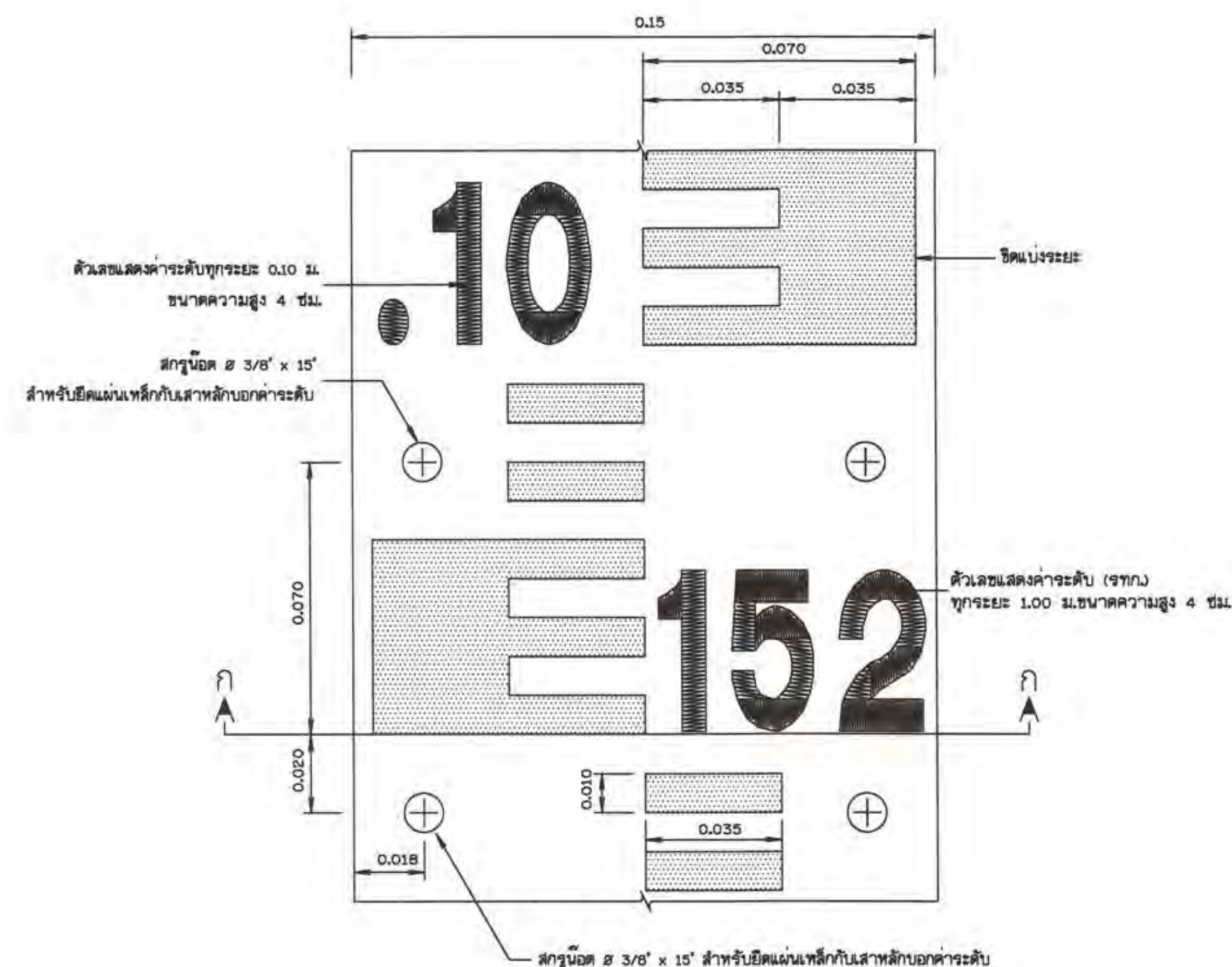
ขยายแผ่นเหล็กบอกระดับน้ำ มาตราส่วน 1:1
