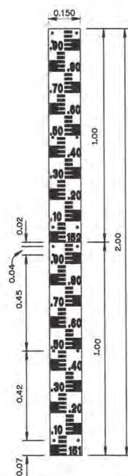
แผ่นเหล็กบอกระดับน้ำ มาตราส่วน 1:10
