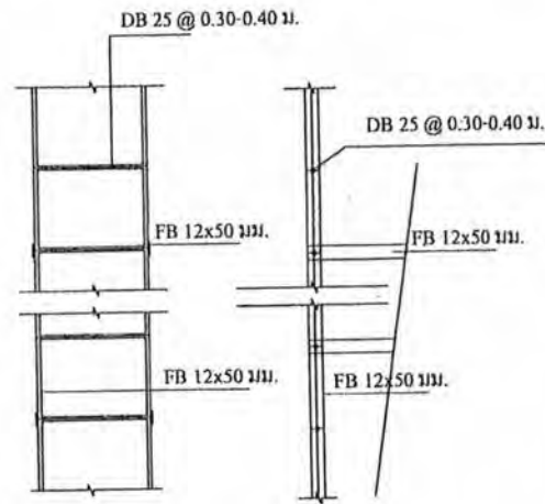
แบบขยายบันได ภายในหม้อหอดังสูง มาตราส่วน 1 : 20
