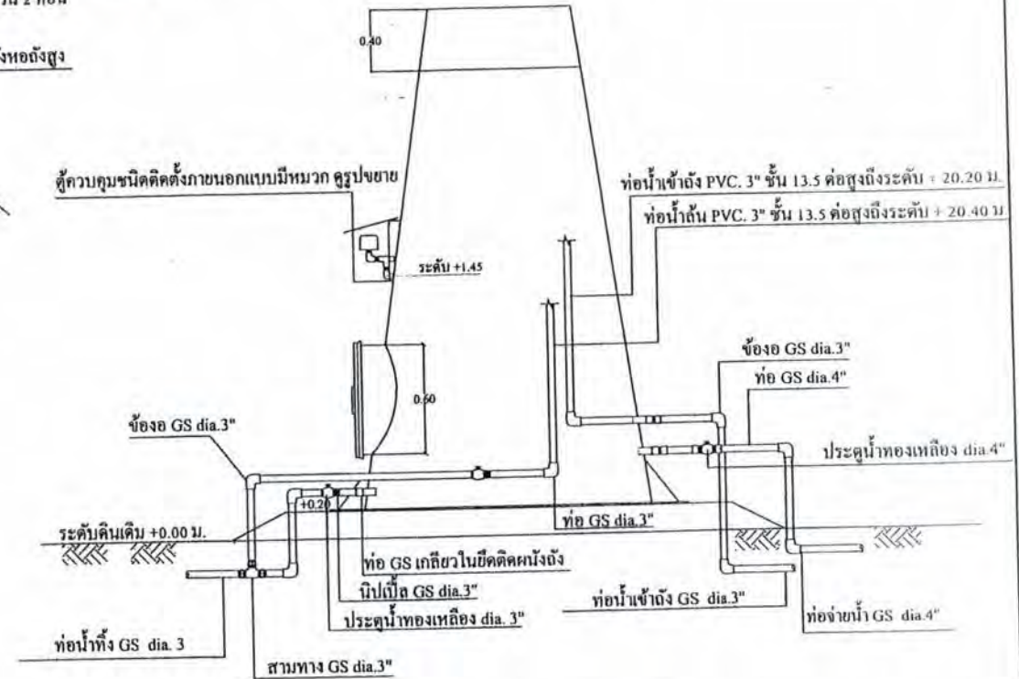
แบบแสดงการเดินท่อในหม้อหอดังสูง มาตราส่วน 1 : 25
