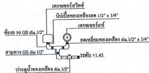
แบบขยายสวิทช์ควบคุมและเกจวัดความดัน
