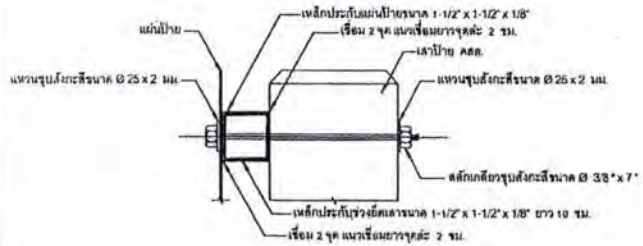
รูปตัดขยายการขีดแผ่นป้ายและเสา มาตราส่วน 1:20
