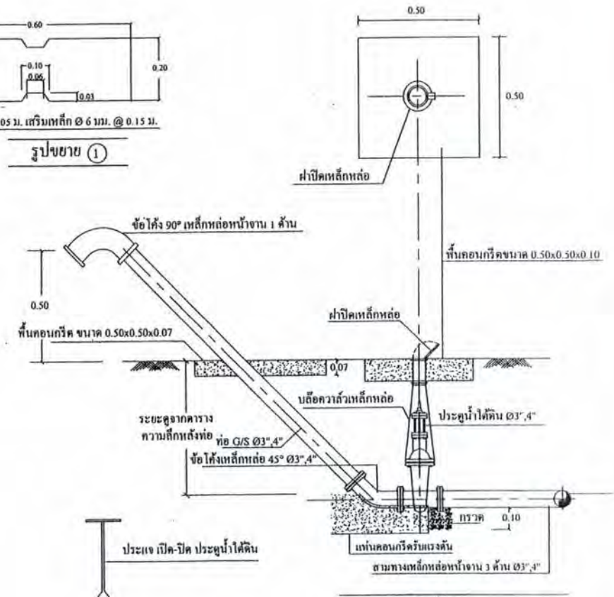
13. แบบการติดตั้งประตูปะทะบวมตะกอน
