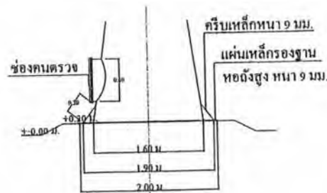
แบบขยายแมนโซลล่างห้องถังสูง มาตราส่วน 1 : 50
