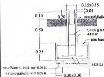
แบบขยายฐานราก F
