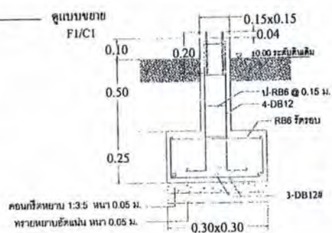
รูปขยายฐานรากโครงสร้างรับแผง FI
