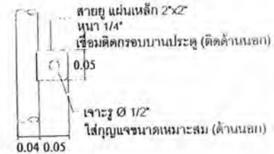
แบบขยายสายยู
