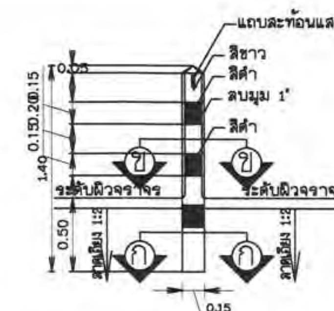
รูปขยายหลักบอกแนว
