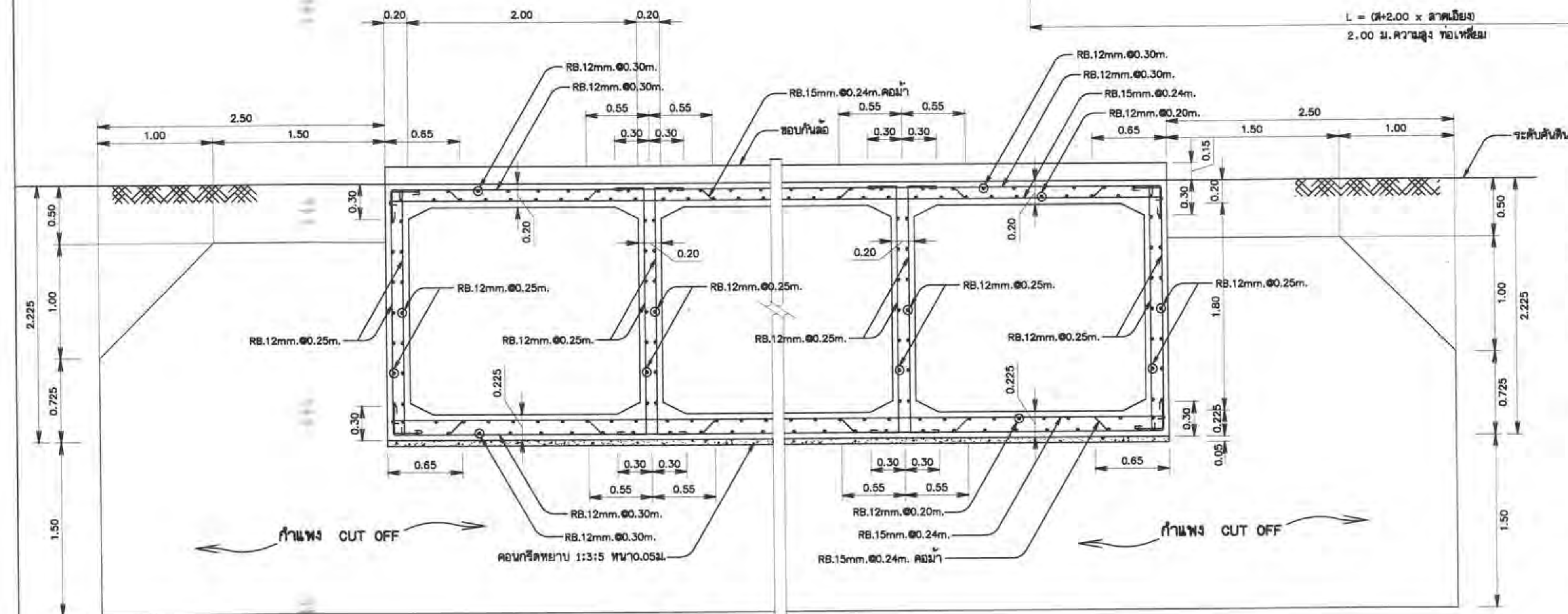
รูปตัด ข - ข มาตราส่วน 1 : 25
