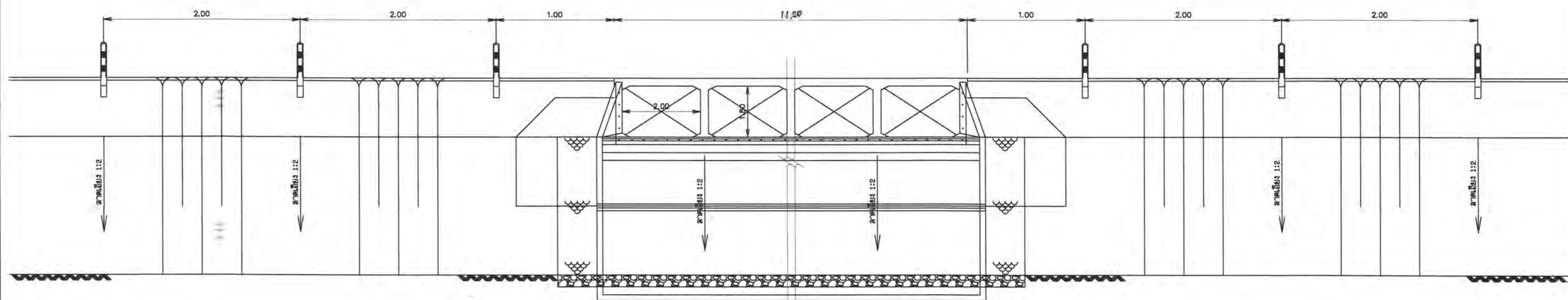
รูปด้านท้ายน้ำ
