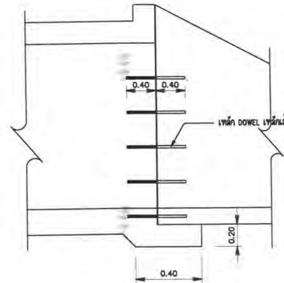
รายละเอียดรอยต่อเพื่อการขยายตัว : ๕/๑
