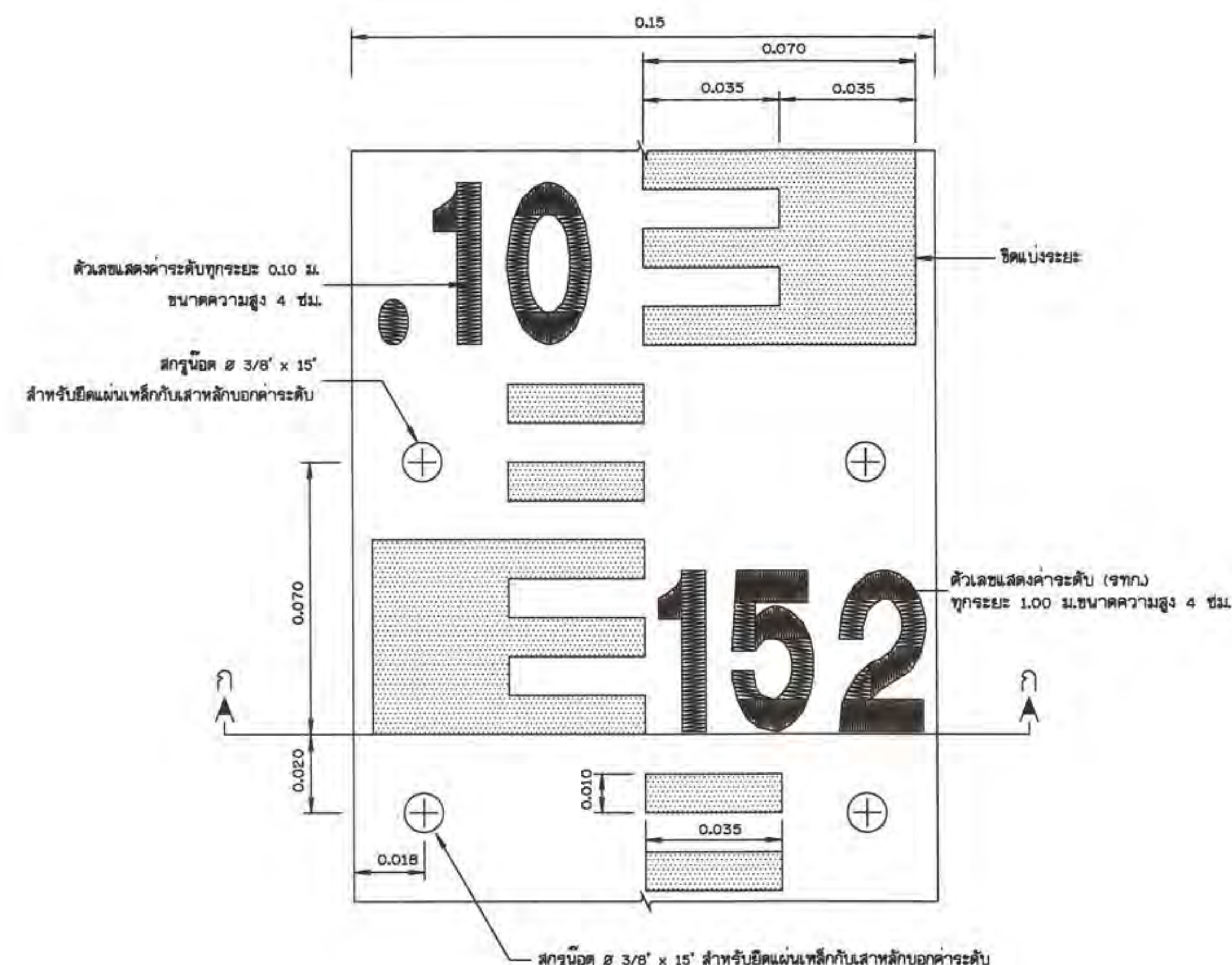
ขยายแผ่นหลักบอกค่าระดับ มาตราส่วน 1:1
