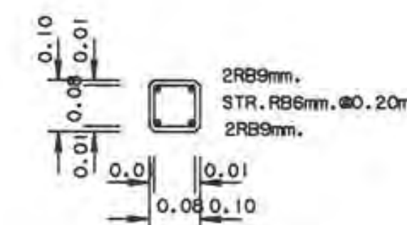
รูปตัด ข - ข
