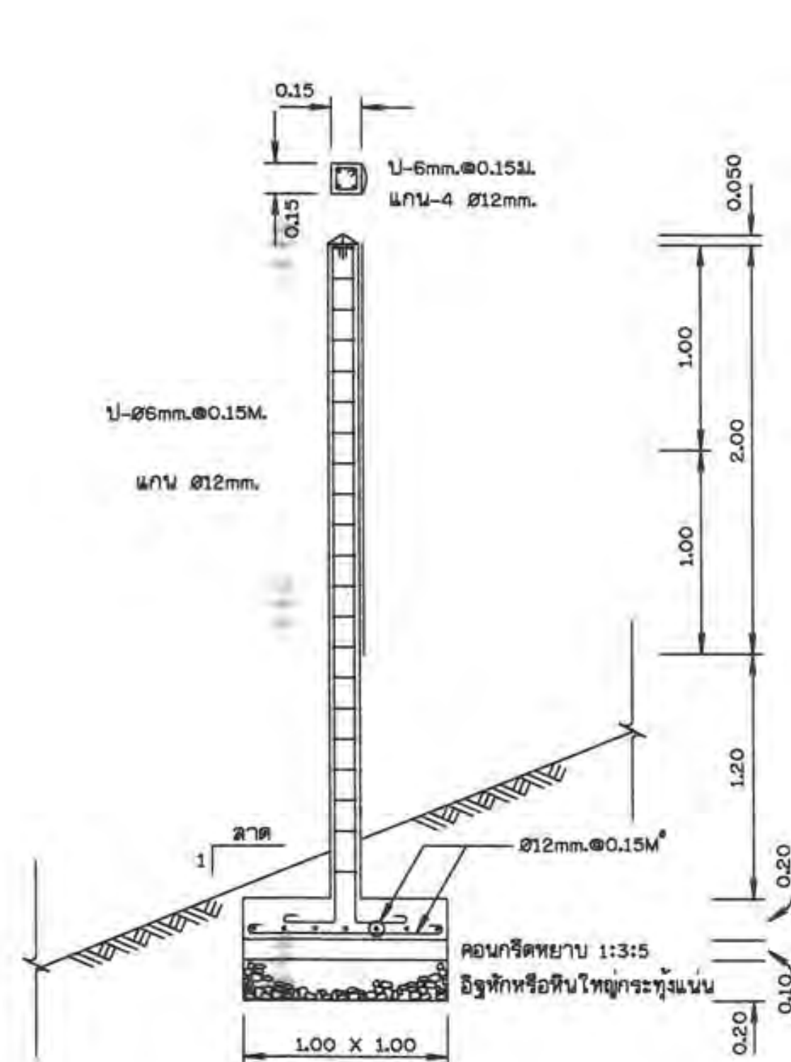
ขยายหลัก คสล.บอกค่าระดับ มาตราส่วน 1:25
