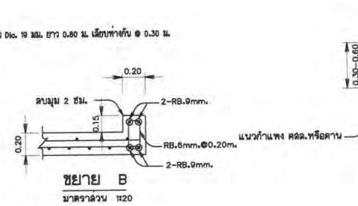
ความกว้างตามแบบแปลน แปลนอาคารระบายน้ำ : ๕/๑
