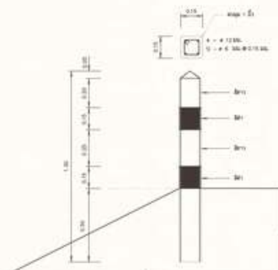
แบบขยายหลักริมคันดิน ขนาดจริง 1:10
