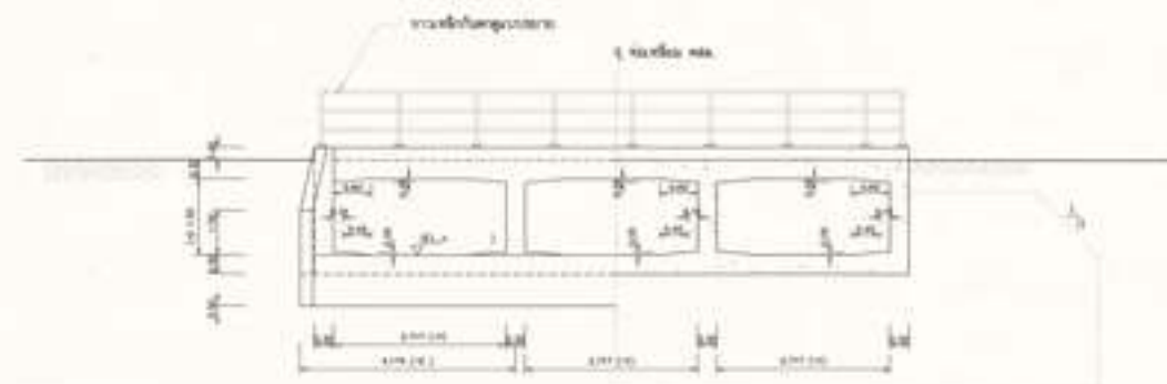
รูปตัด C - C
