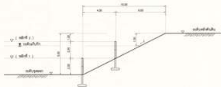
รูปตัดหัวไปแสดงตำแหน่งหลักบอกค่าระดับน้ำ
