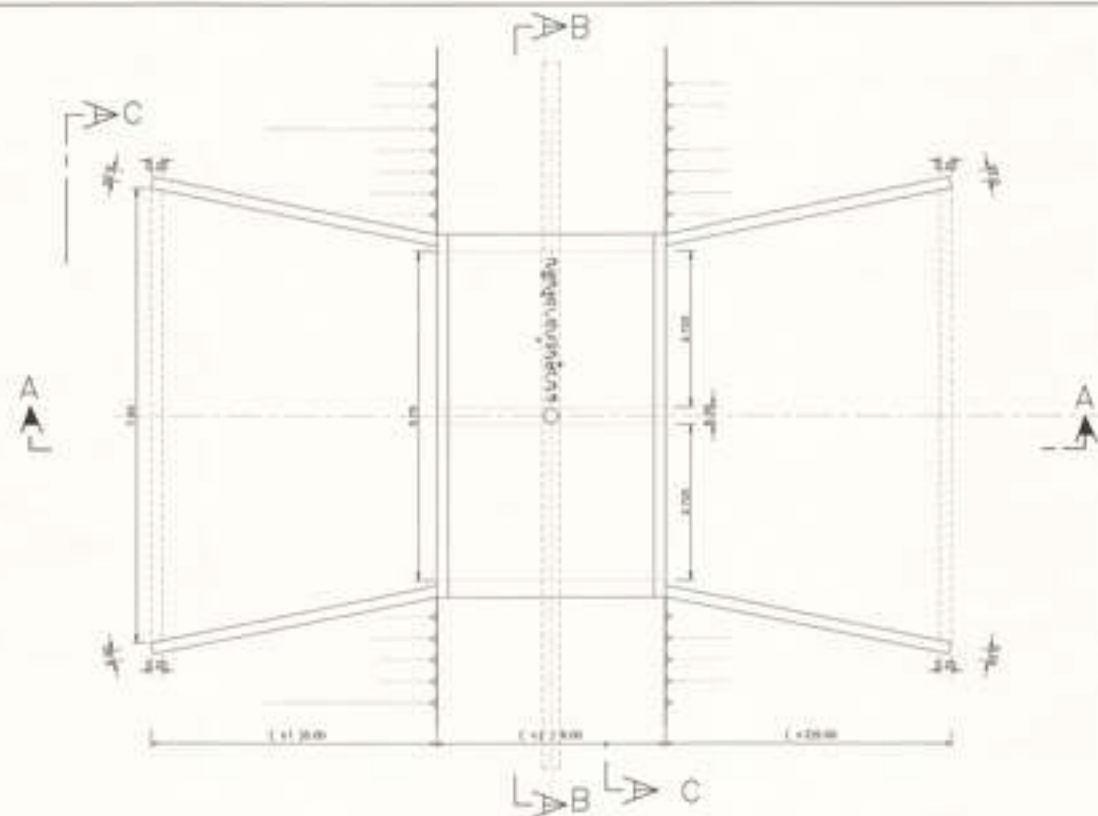
แปลนอาคารระบายน้ำ ขนาดจริง 1:50
