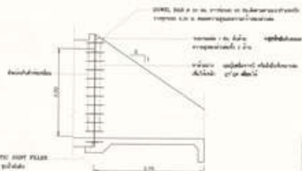
แบบแสดงรอยต่อระหว่างท่อกับปีกกำแพง
