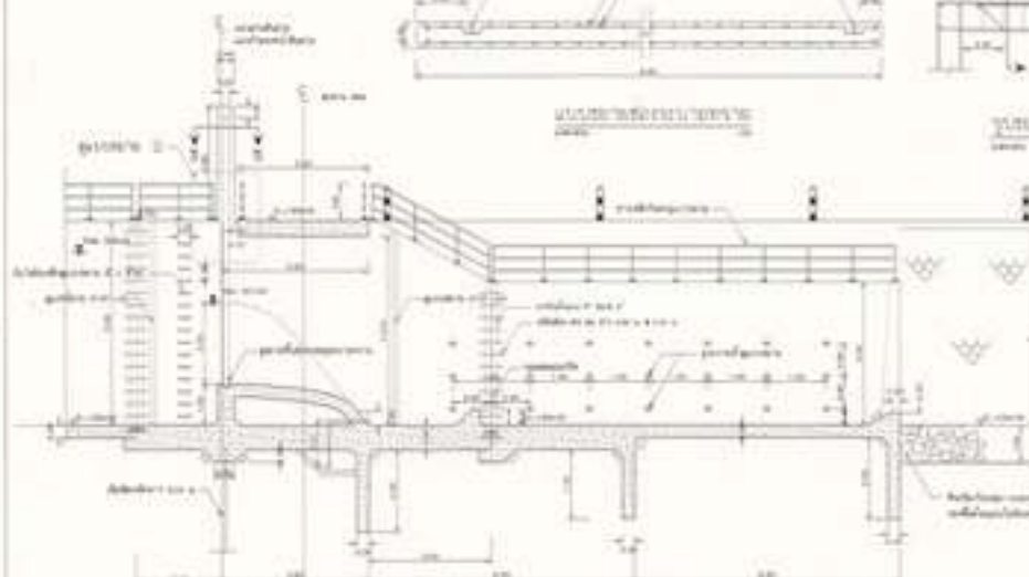
มุมมองด้านหน้า หน้า
