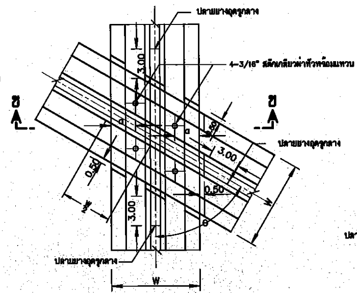
การต่อพาดทับกันไม่ทำมุมฉาก ไม่แสดงมาตรฐาน
