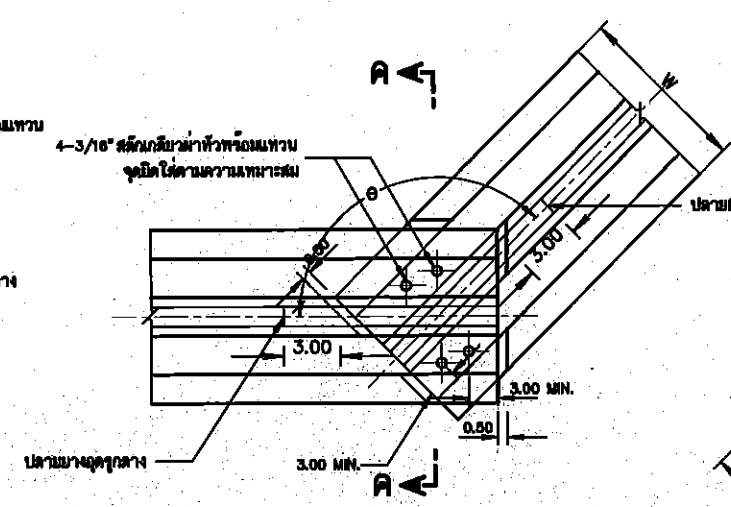
การต่อทำมุมกัน ไม่แสดงมาตรฐาน
