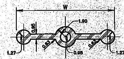
TYPE 'A' ไม่แสดงมาตรฐาน
