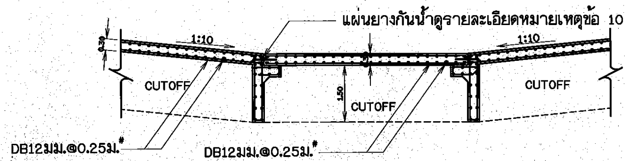
แบบขยาย 3
