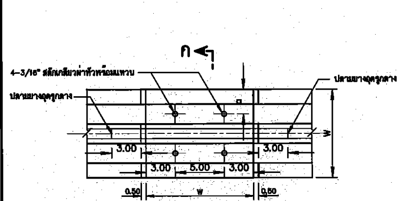
การต่อตรง ไม่แสดงมาตรฐาน
