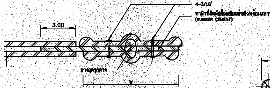
รูปตัด ง-ง ไม่แสดงมาตรฐาน
