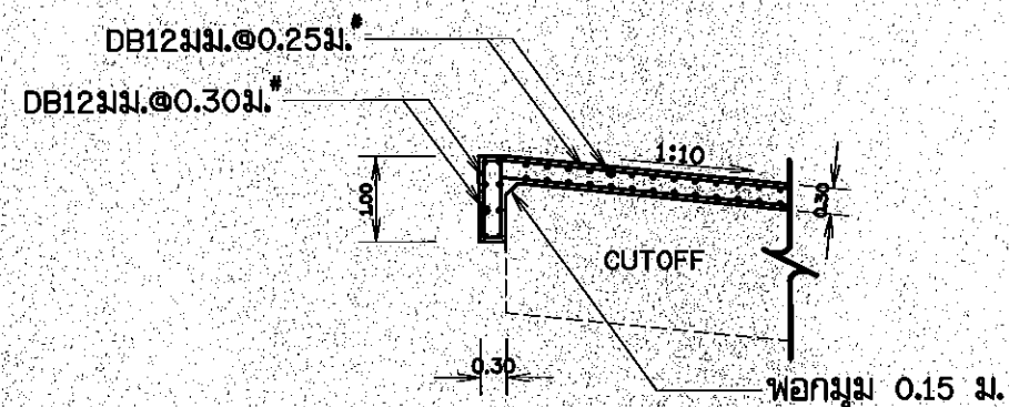
แบบขยาย 4
