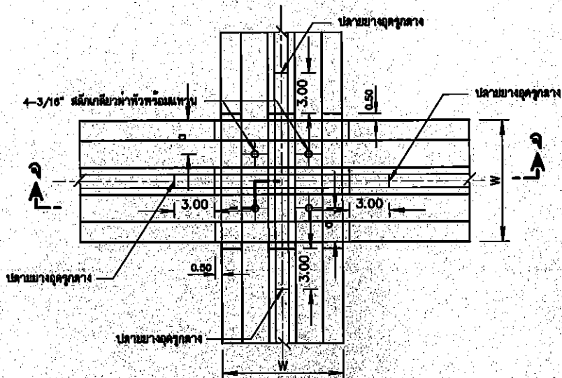
การต่อพาดทับกันทำมุมฉาก ไม่แสดงมาตรฐาน
