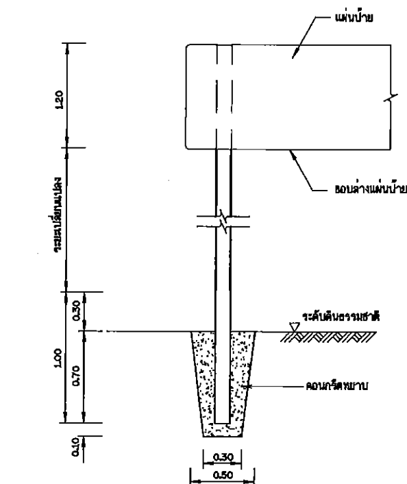
รายละเอียดการติดตั้งเสาป้าย
