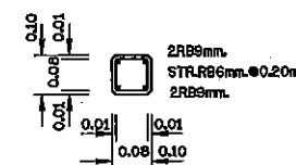
รูปตัด ข - ข มาตรฐาน 1:10
