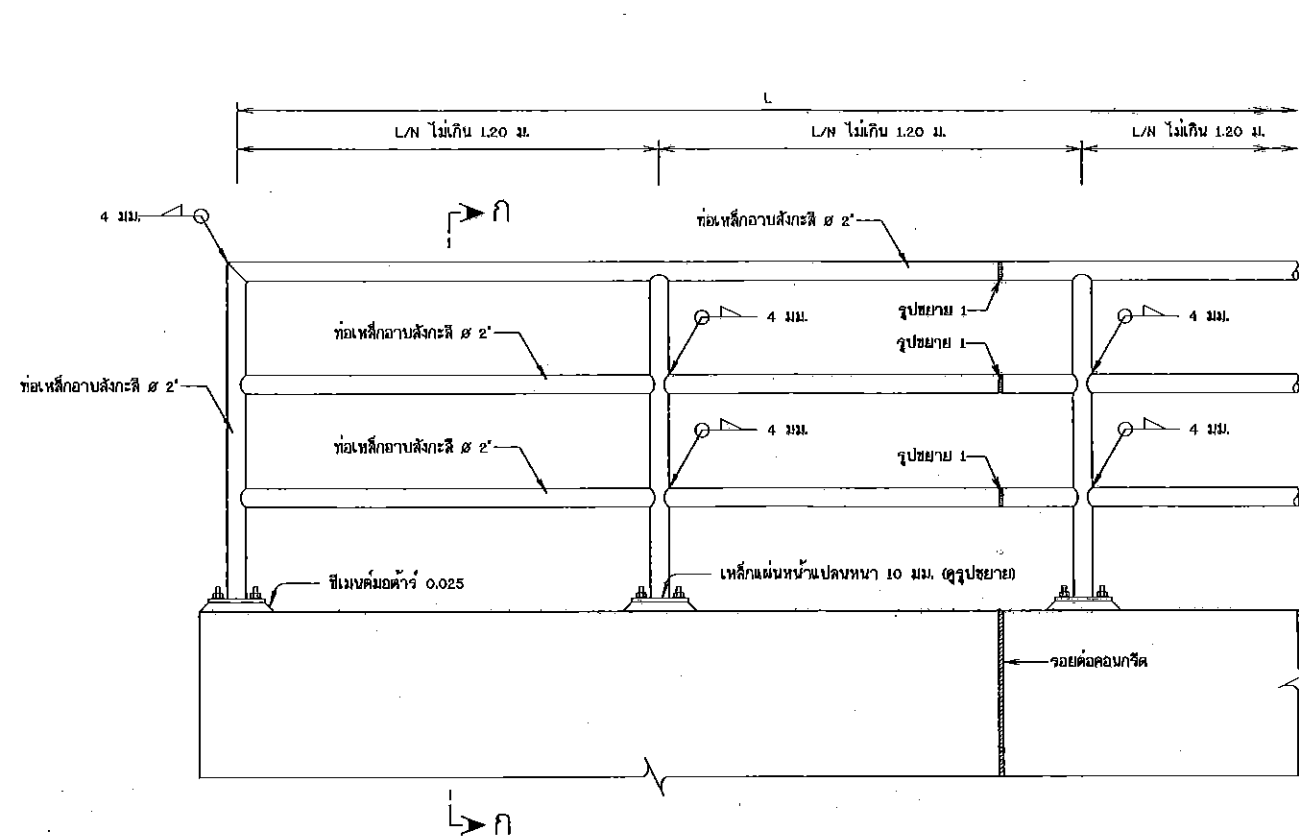
รูปขยายจาวเหล็กกันตก
