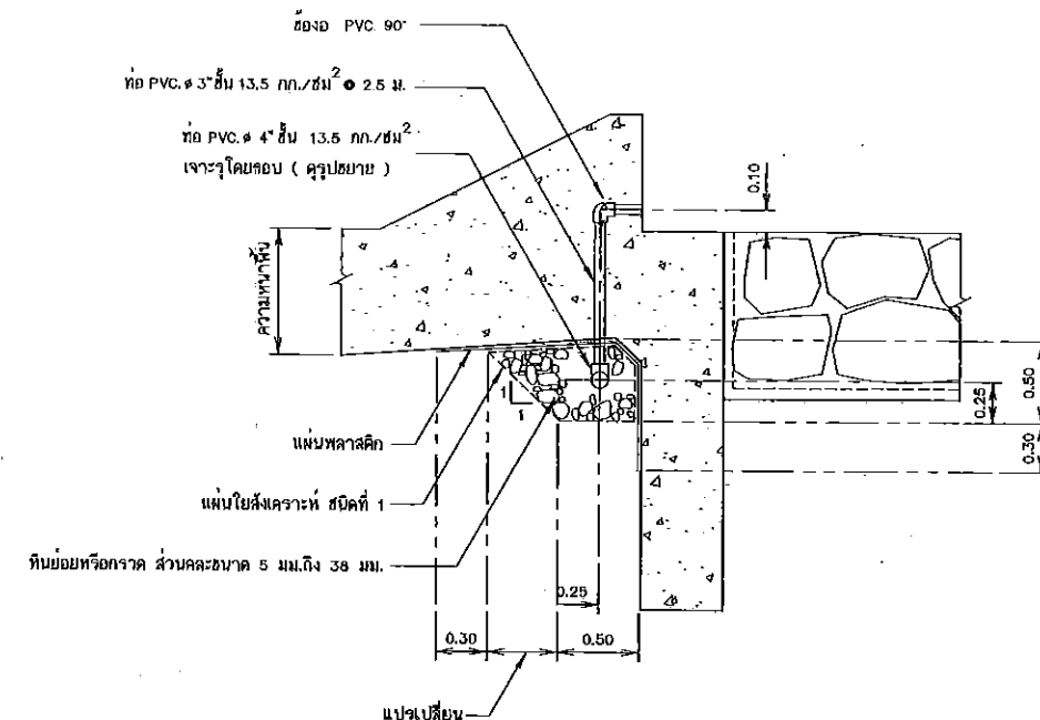
รูปขยายระบายน้ำใต้อาคาร แบบที่ 3
