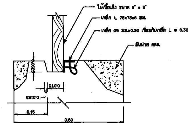
แบบขยาย 3 มาตราส่วน 1:15
