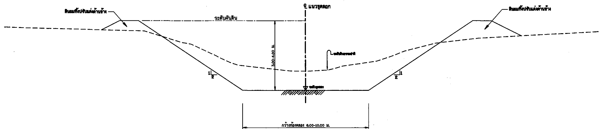
รูปตัดทั่วไปแสดงการขุดลอก
