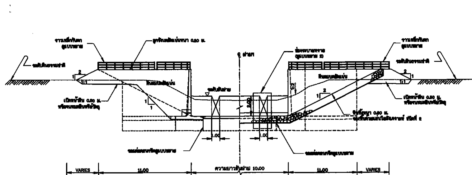
รูปตัด ค-ค มาตราส่วน 1:125
