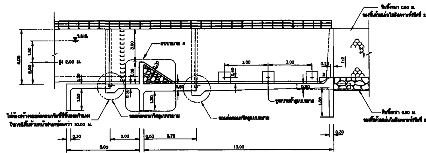
รูปขยาย 1 มาตราส่วน 1:75
