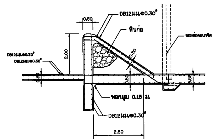
แบบขยาย 4 มาตราส่วน 1:80
