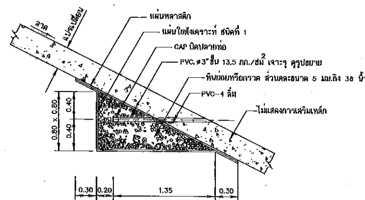
รูปขยายระบายน้ำกำแพงลาดเอียง
