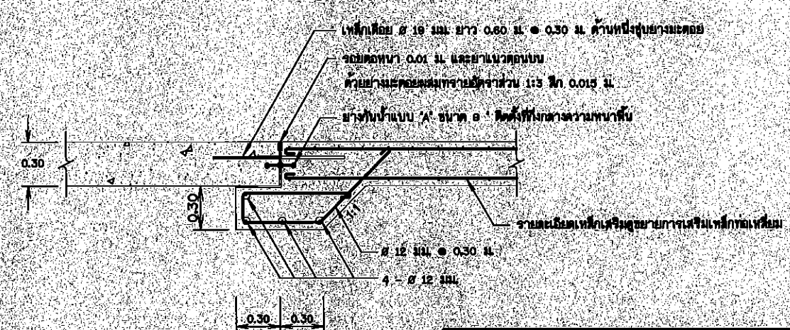
รูปขยายรอยต่อคอนกรีต
