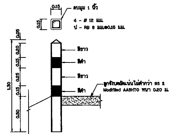
แบบขยายหลักกันดก คสล.
