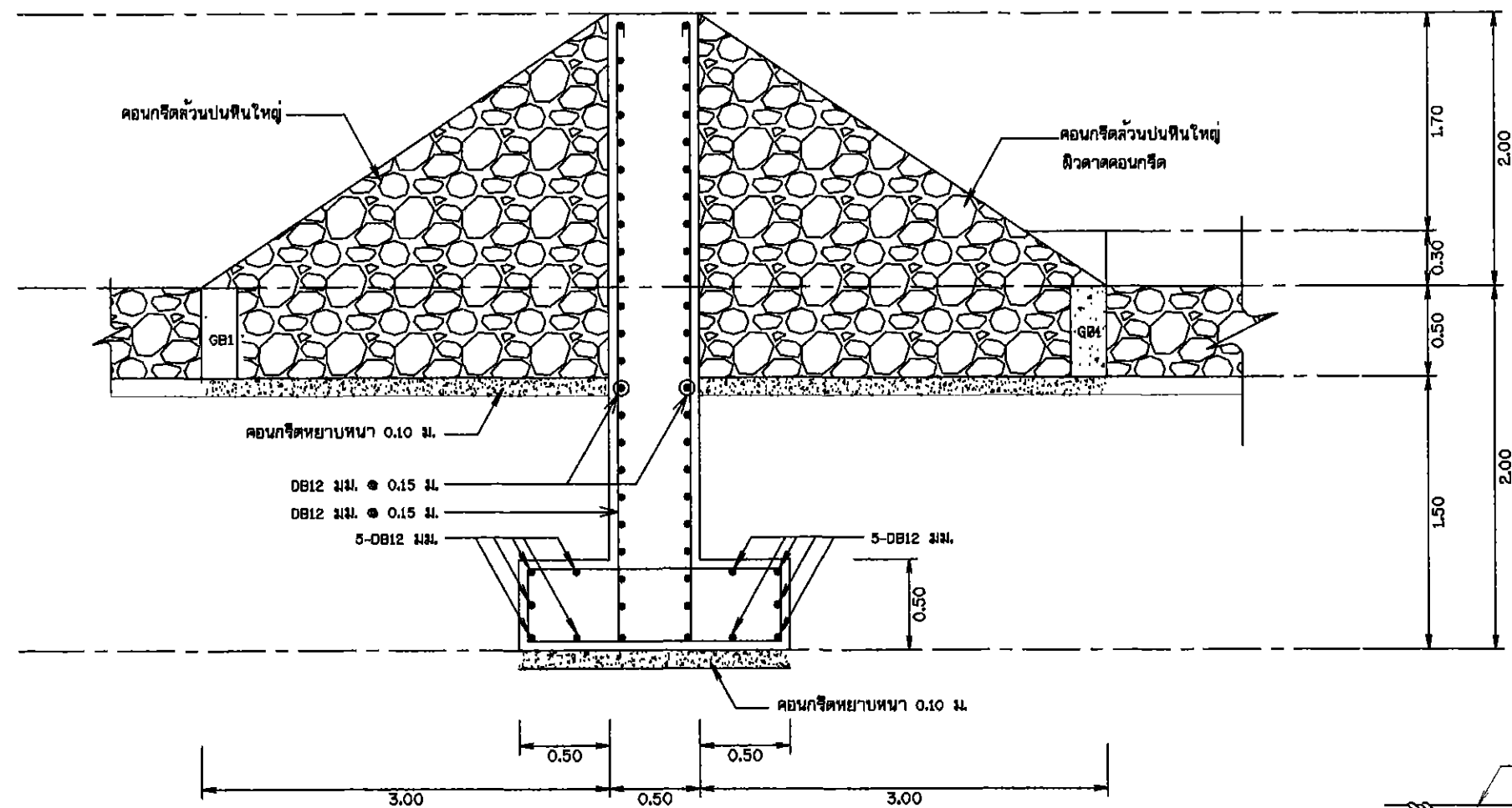
รูปตัดแสดงการเสริมเหล็กแกนฝ่ายๆ
