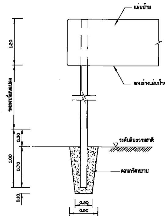
รายละเอียดการติดตั้งเสาป้าย ขนาด: 1:20
