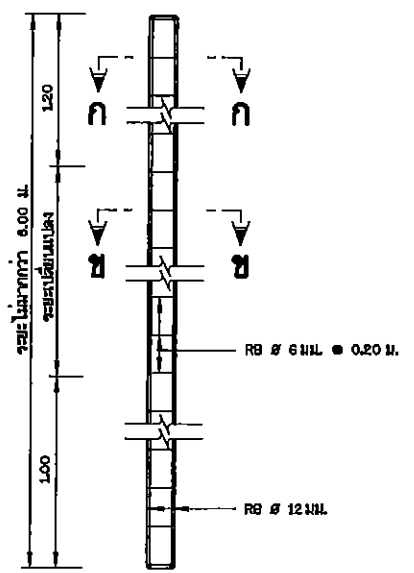
รายละเอียดเสาป้าย คสล. ขนาด: 1:20
