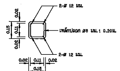
รูปตัด ข - ข ขนาด: 1:10
