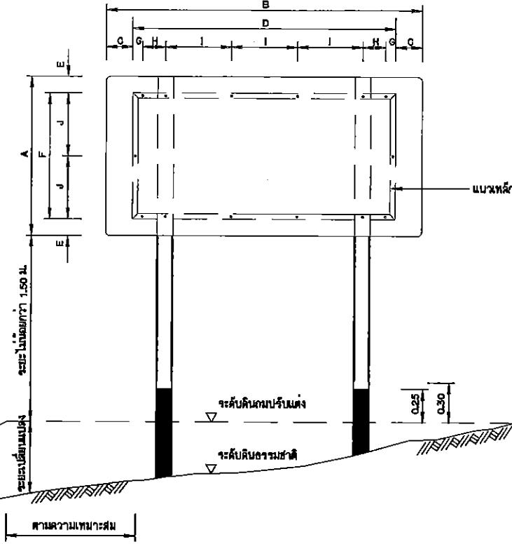
รูปแสดงการประกอบแผ่นป้าย ขนาด: 1:20
