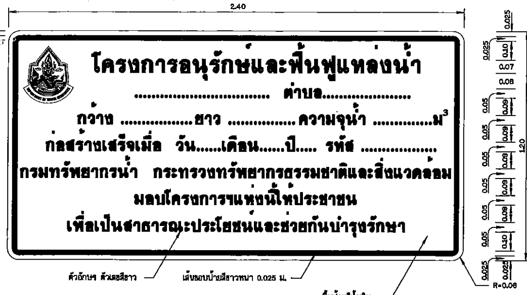
ป้ายโครงการ ขนาด: 1:10
