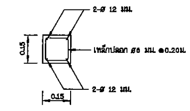
รูปตัด ก - ก ขนาด: 1:10
