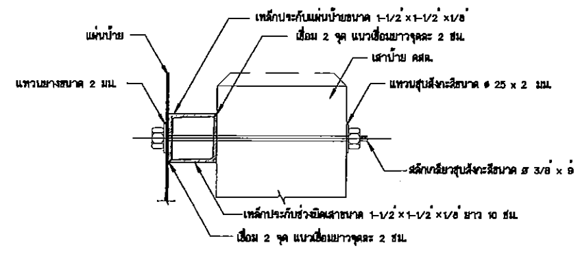
รูปตัดขยายการยึดแผ่นป้ายและเสา ขนาด: 1:20
