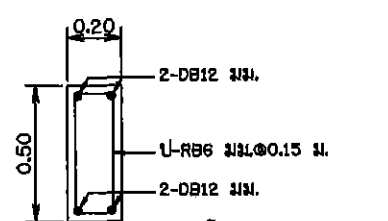
ขยายคานคอดิน GB1
