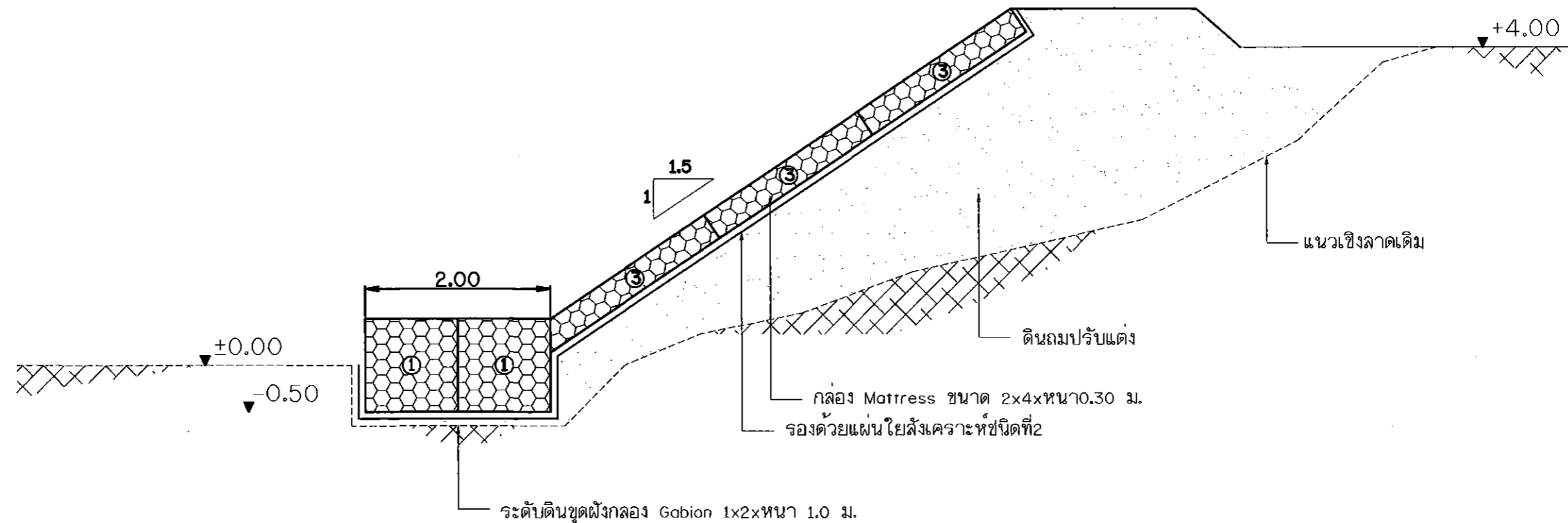
ป้องกันการกัดเซาะริมตลิ่งแบบวางเรียงด้วยเกเบียนและแมทเทรลส์ กรณีปรับความลาดชันของผิวหน้าเชิงลาดเท่ากับ 1:2 มาตรฐาน 1:50
