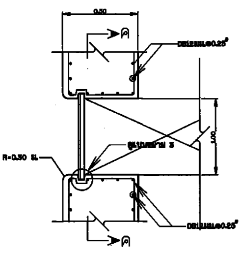
แบบแปลนช่องระบายน้ำ มาตราส่วน 1:25
