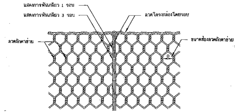
รูปแสดงการพันลวดระหว่างกล่องลวดตาข่ายและผ้าปิด
