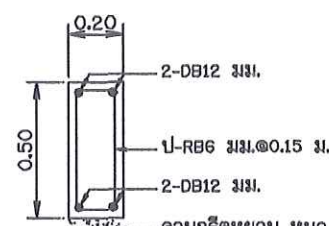
ขยายคานคอดิน GB1
