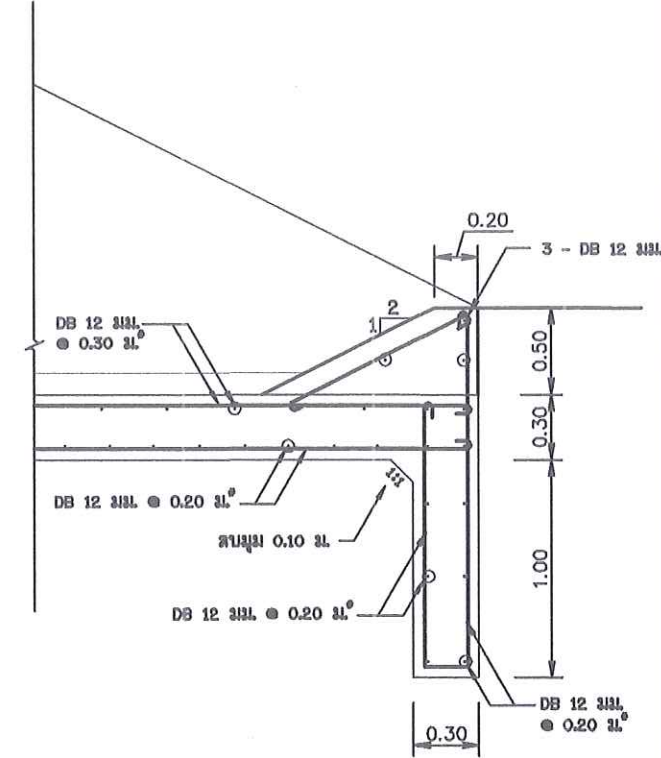
แบบขยาย " 2 "
