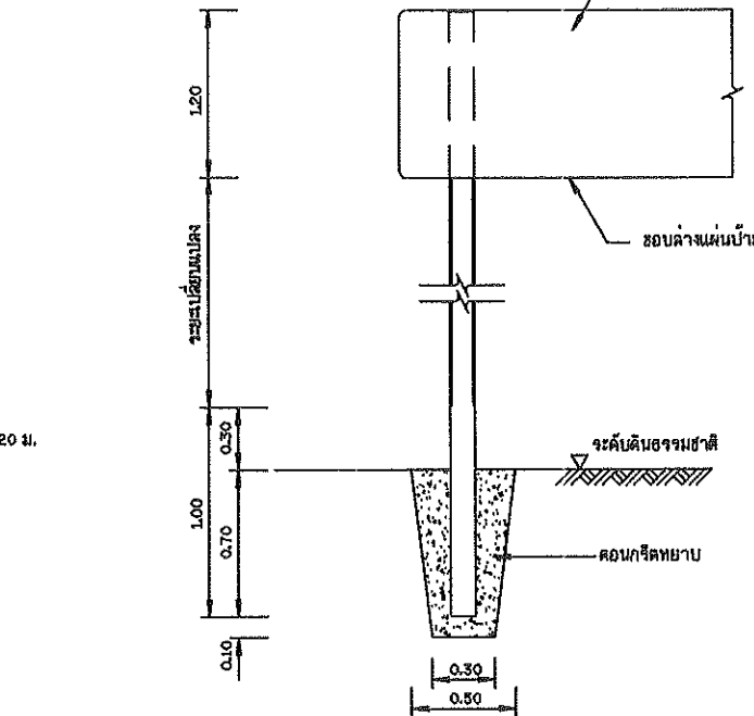
รายละเอียดการติดตั้งเสาป้าย
