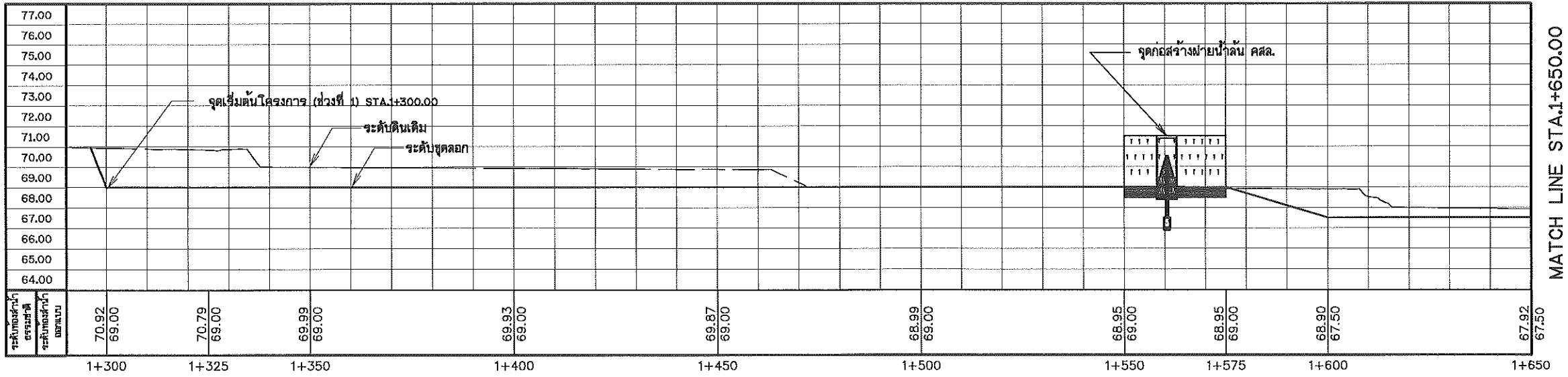
รูปตัดตามยาวแสดงการขุดลอก ช่วงที่ 2 มาตราส่วน 1:250 แนวนอน 1:500
