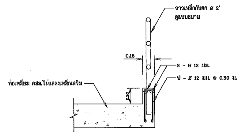
รูปขยาย 1
