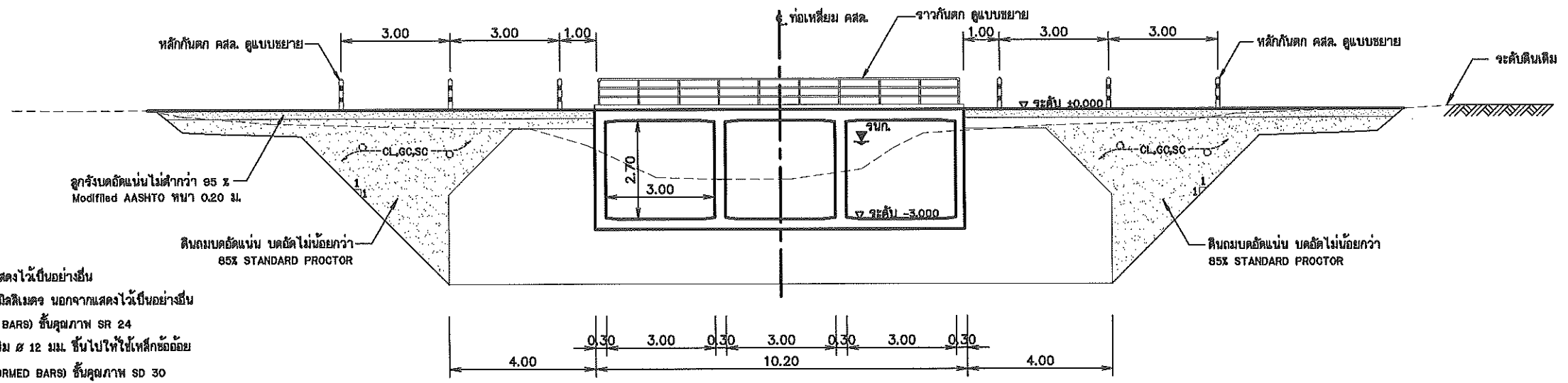
รูปตัดตามขวางแนว ข - ข มาตราส่วน 1:100
