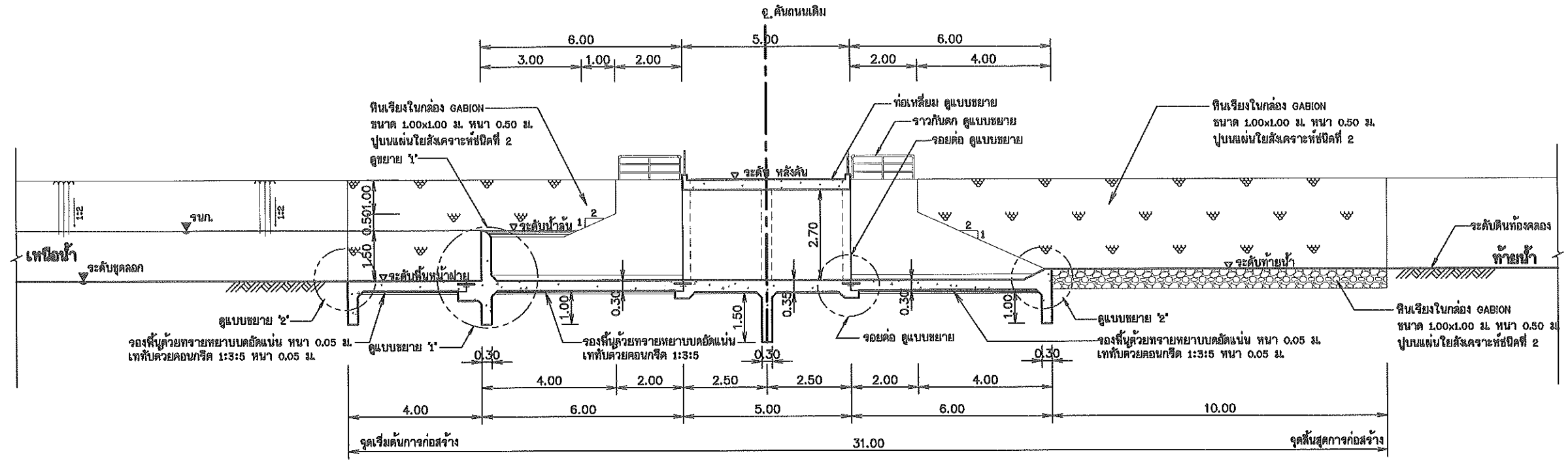
รูปตัดตามยาวแนว ก - ก มาตราส่วน 1:100
