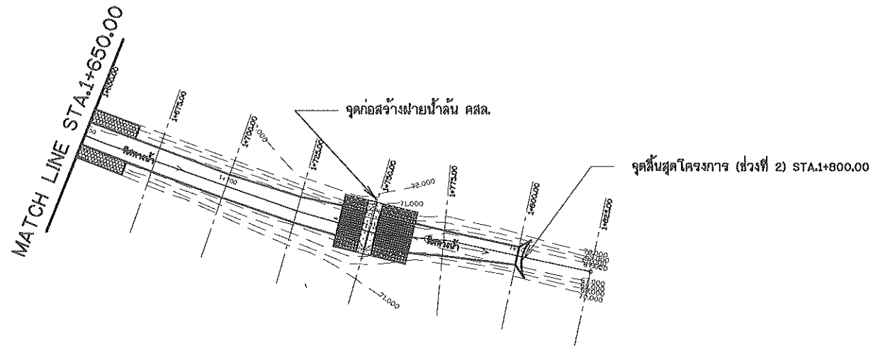
แปลนแสดงการขุดลอก ช่วงที่ 2 มาตราส่วน 1:1000
