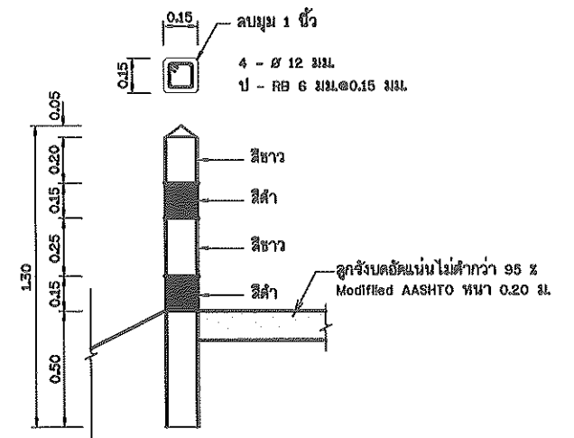
แบบขยายหลักกันคก คสล.
