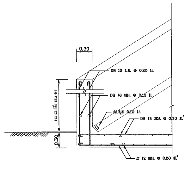
รูปตัด "ง"
