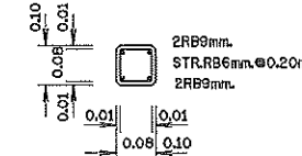
รูปตัด ข - ข
