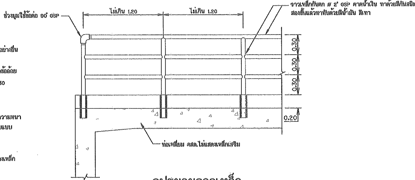
รูปขยายราวเหล็ก
