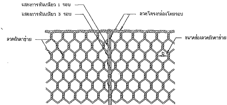
รูปแสดงการพันลวดระหว่างกล่องลวดตาข่ายและฟาปิด
