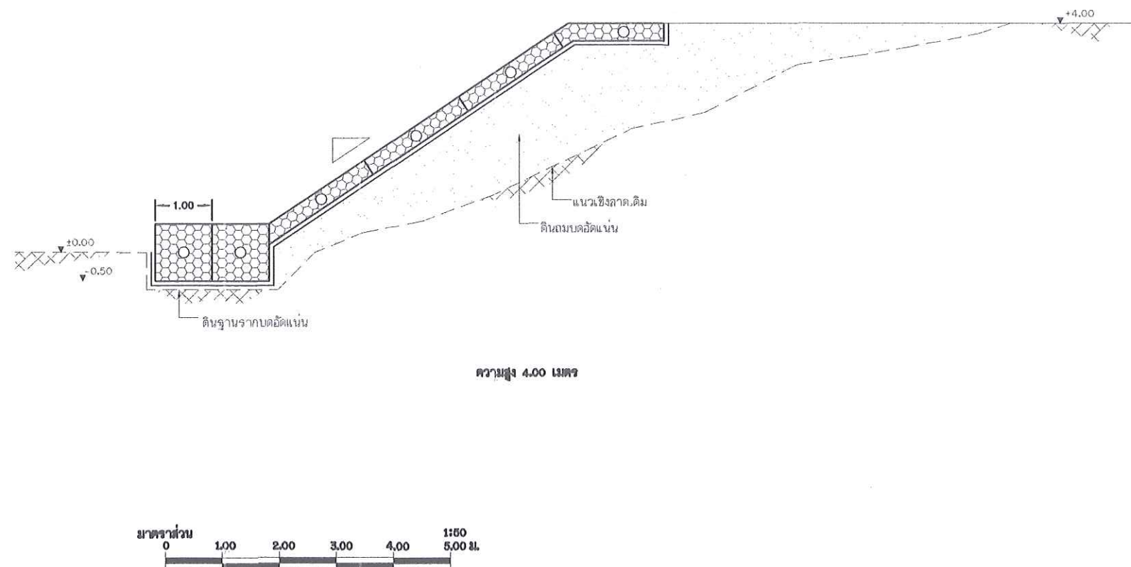
ระบบป้องกันการกัดเซาะริมตลิ่งแบบวางเรียงด้วยเกเบียนและแมทเทรล กรณีปรับความลาดชันของผิวหน้าเชิงลาดเท่ากับ 1:1.5 (ตั้ง : ราบ) รูปแบบที่ 1
