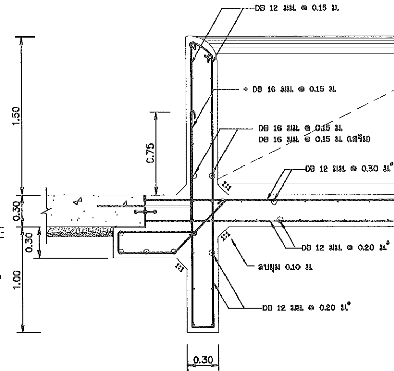
แบบขยาย " 1 "
