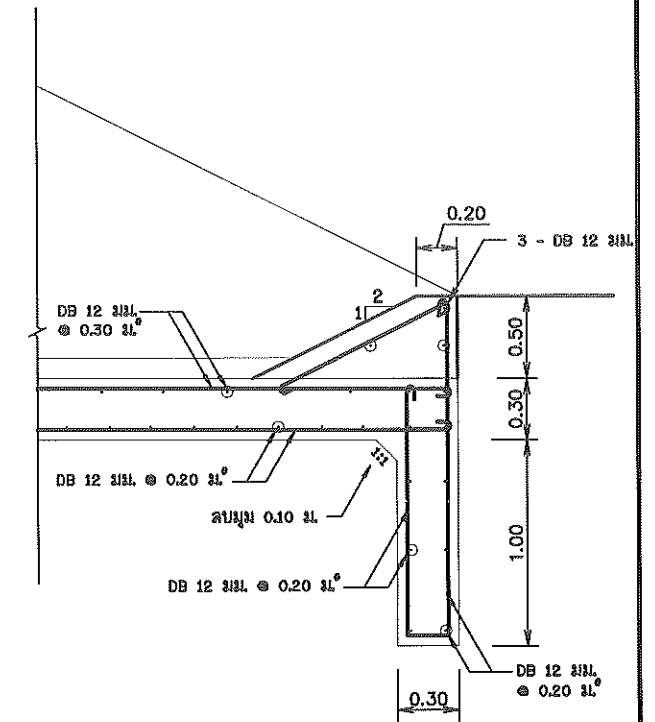
แบบขยาย " 2 "
