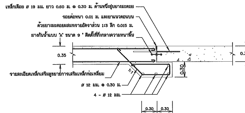
รูปขยายรอยต่อคอนกรีต
