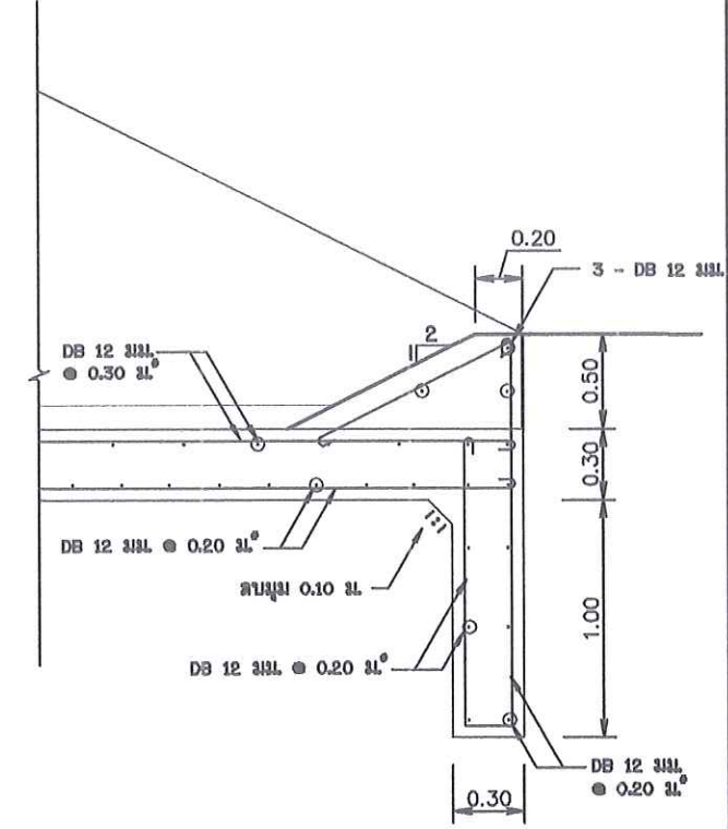
แบบขยาย " 3 "
