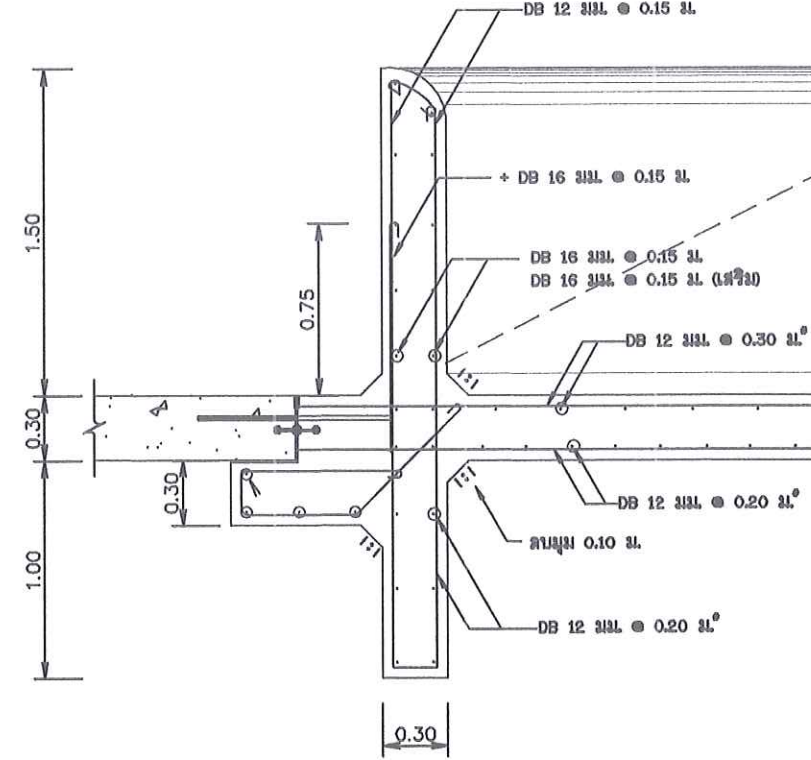
แบบขยาย " 1 "
