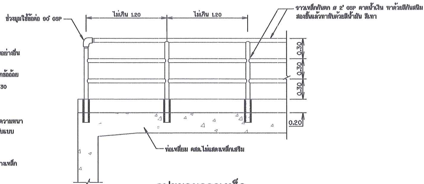
รูปขยายจาวเหล็ก
