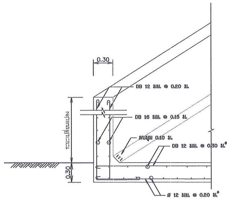
รูปตัด "ง"
