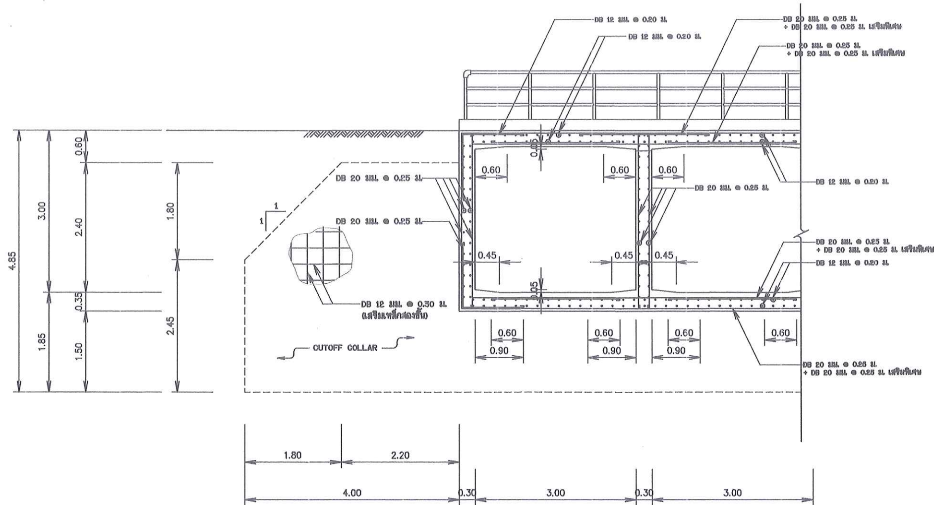
รูปตัดขยายการเสริมเหล็ก
