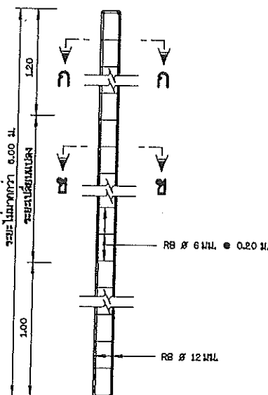
รายละเอียดเสาป้าย คสล. 1:20
