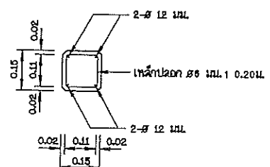
รูปตัด ข - ข 1:10
