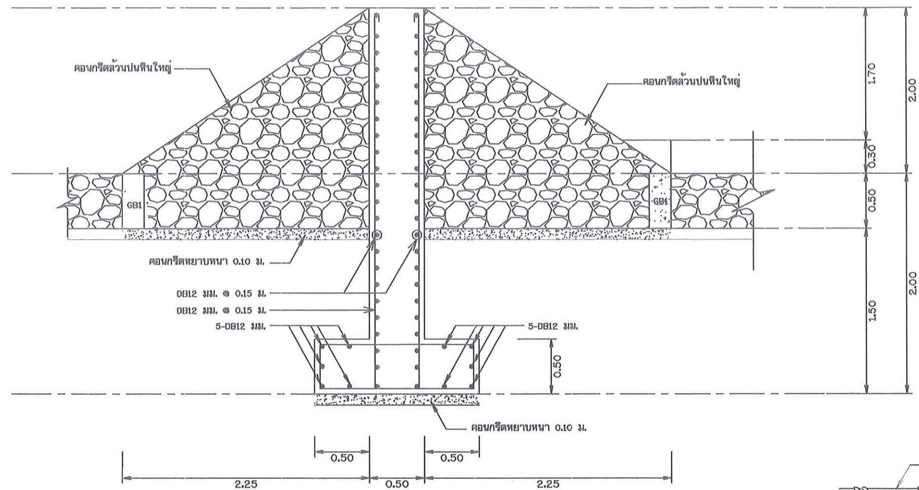
รูปตัดแสดงการเสริมเหล็กแกนฝายฯ
