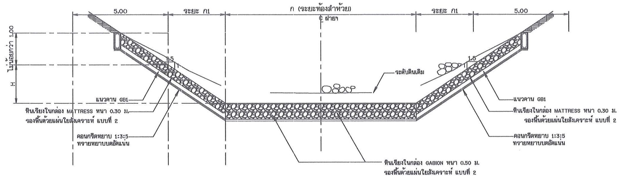
รูปตัด ค-ค
