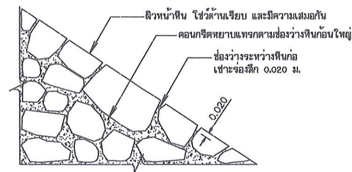
ขยายคอนกรีตล้นบนพื้นใหญ่
