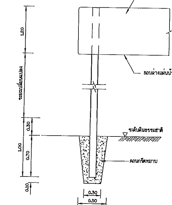
รายละเอียดการติดตั้งเสาป้าย 1:20
