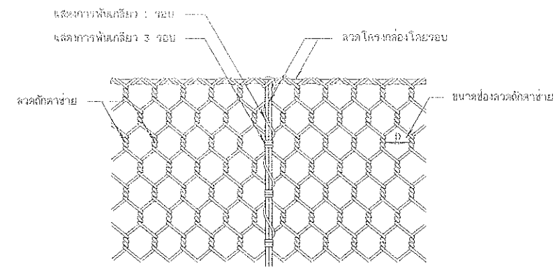
รูปแสดงการผันลดระหว่างกล่องลดตาข่ายและฝาปิด
