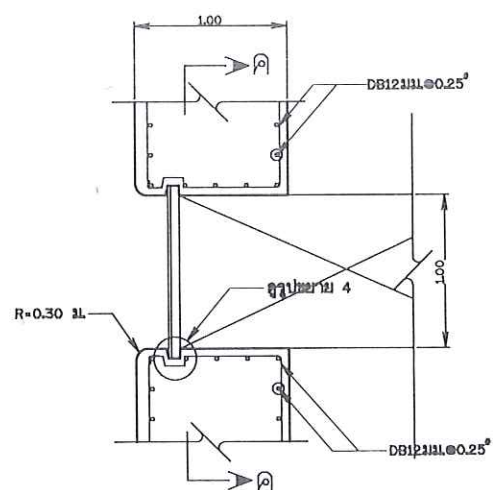
รูปขยายช่องระบายทราย มาตราส่วน 1:25
