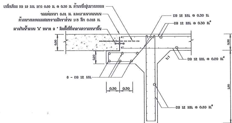
รูปขยายรอยต่อคานกรีต มาตราส่วน 1:20
