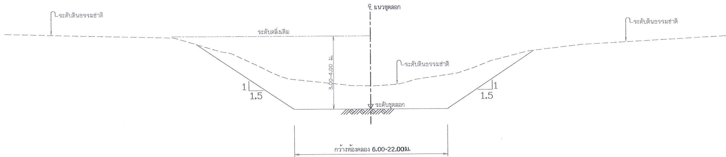
รูปตัดทั่วไปแสดงการขุดลอก มาตราส่วน ไม่ระบุ
