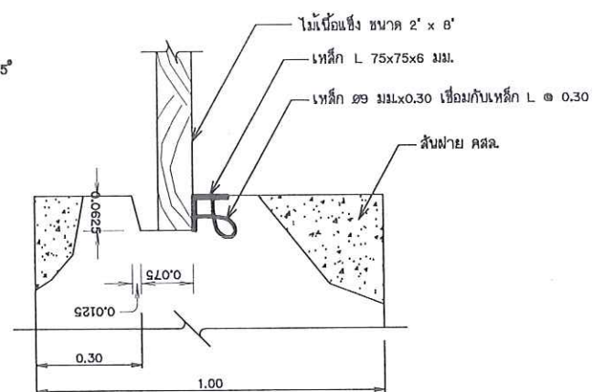
รูปขยาย 4 มาตราส่วน 1:5
