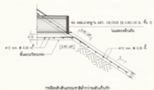
กรณีดินถมถมหน้าท่อตันกับดิน
