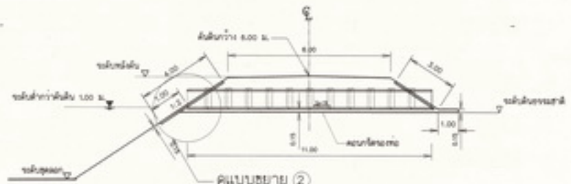
SECTION D - D ขนาดจริง 1 : 100
