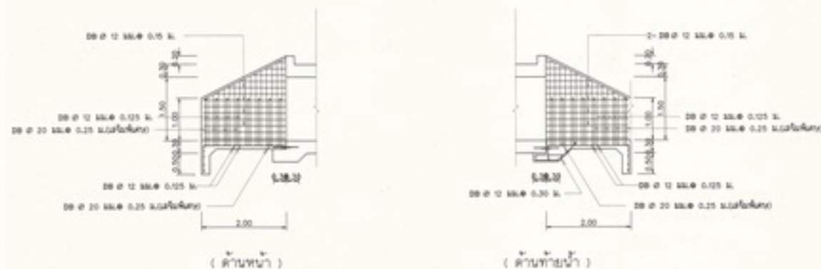
รูปตัดขยายการเสริมเหล็กแนว 3 - 3
