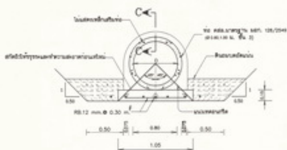
รูปตัดพื้นรองท่อ คล. 1 แถว ขนาดจริง 1 : 25
