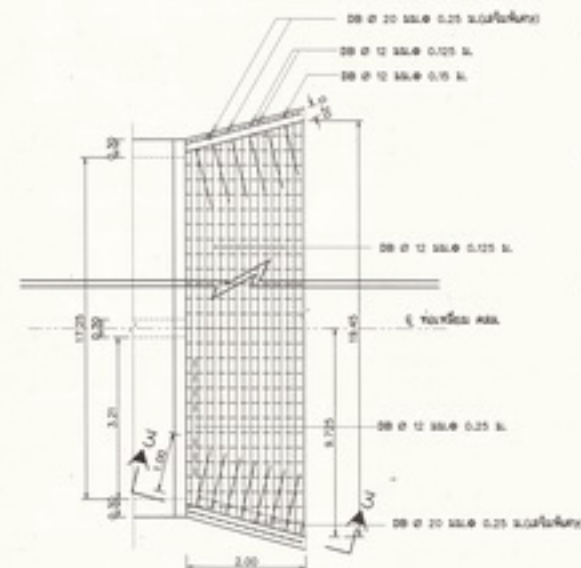
แสดงการเสริมเหล็กปากท่อเหลี่ยม คสล.
