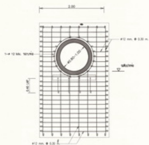
แบบขยายเหล็กเสริมคอนกรีตปากท่อตันใน ขนาดจริง 1 : 25
