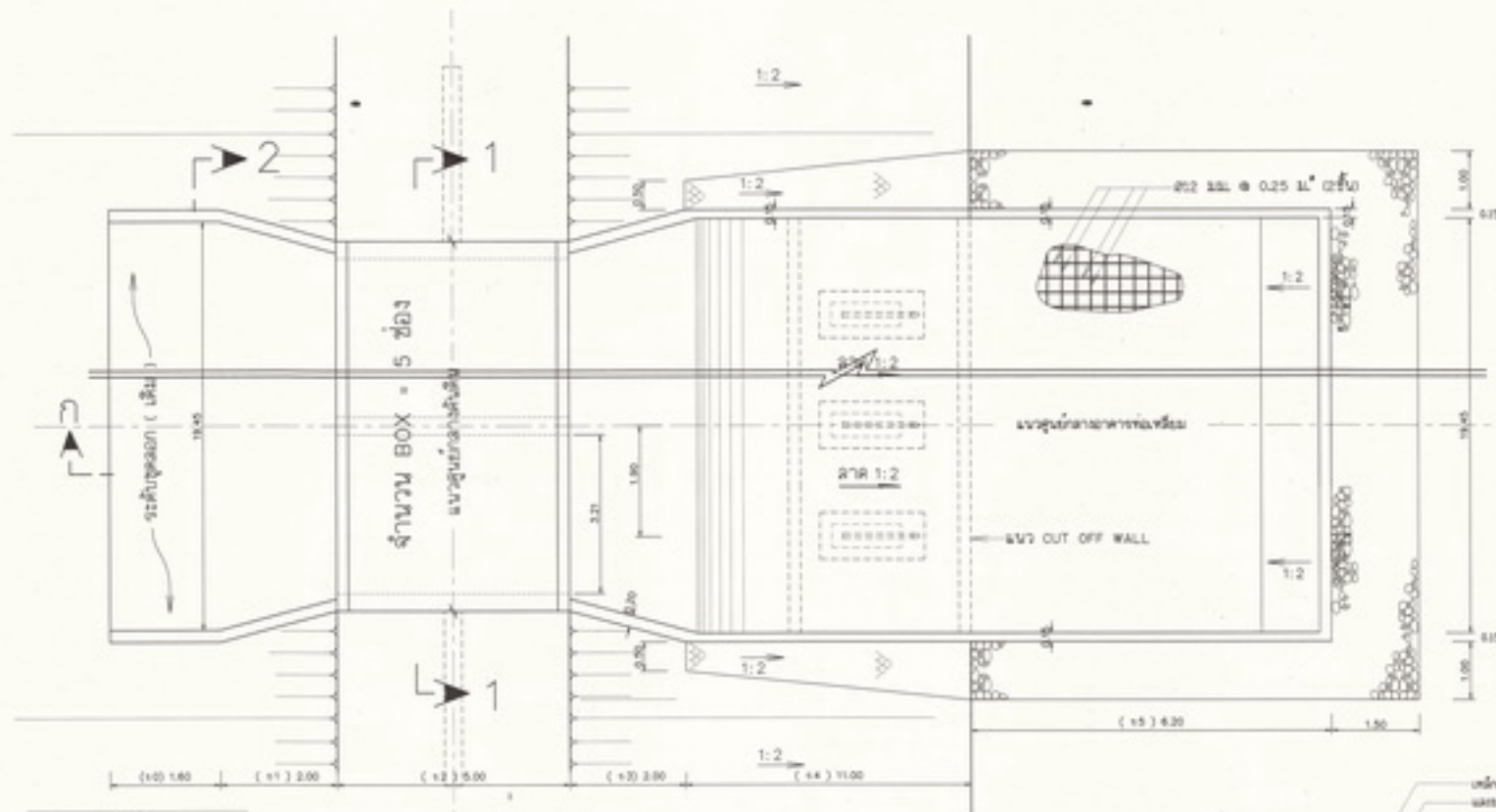
แปลนอาคารระบายน้ำ มาตราส่วน 1:50
