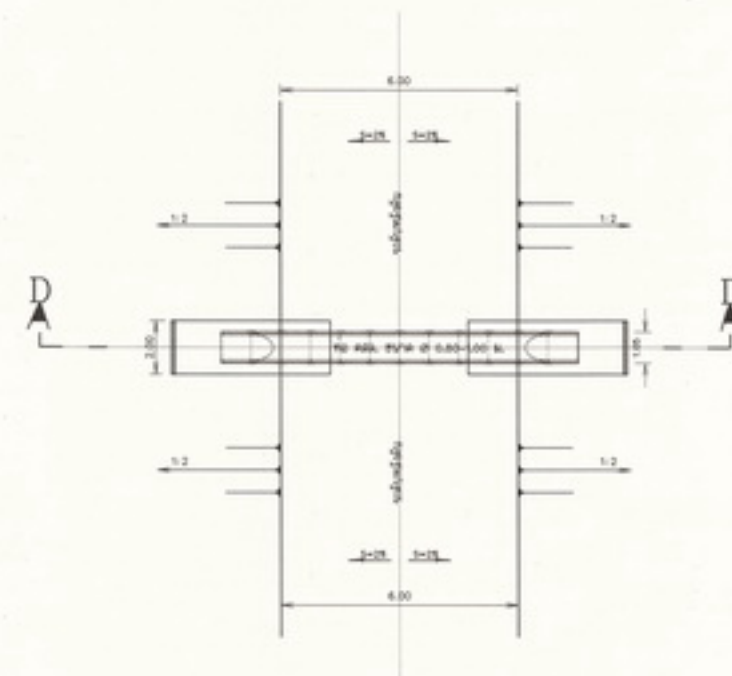
แปลนอาคารระบายน้ำออก ขนาดจริง 1 : 100
