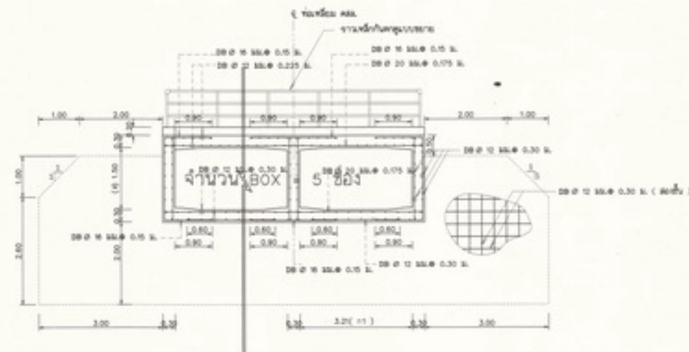
รูปตัดขยายการเสริมเหล็กแนว 1 - 1
