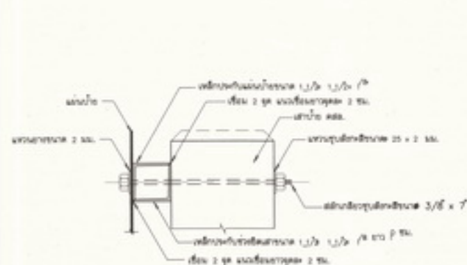
รูปตัดขยายการยึดแผ่นป้ายและเสา มาตราส่วน 1:3
