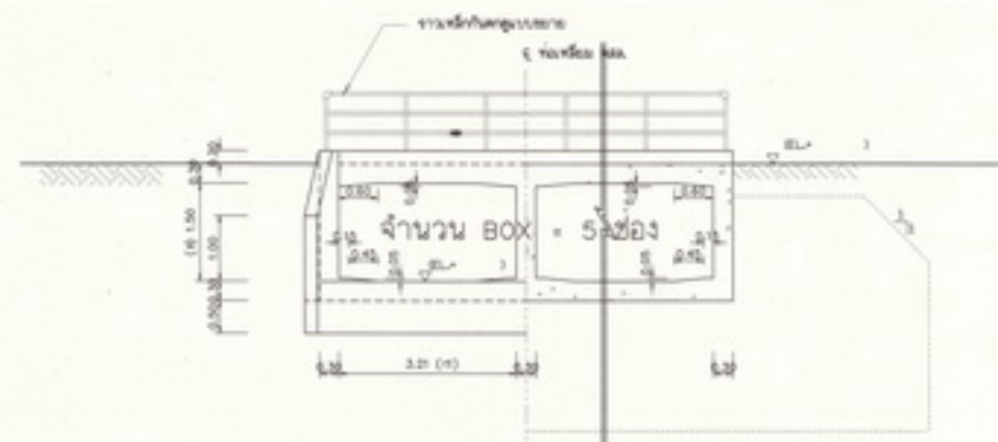
รูปตัด 2 - 2
