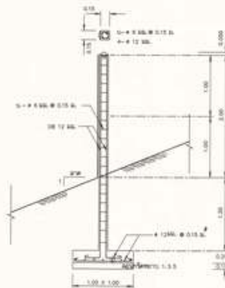
ขยายหลัก คสล. แสดงค่าระดับ ขนาดจริง 1:25
