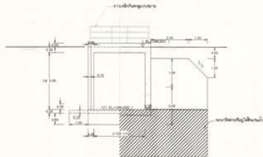
รูปตัด C - C
