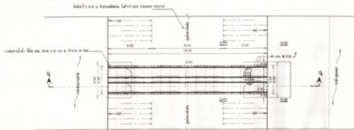
แปลนวางท่อ คล.ล. ขนาดจริง 1 : 100
