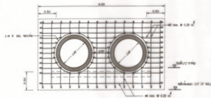
แบบขยายเหล็กเสริมคอนกรีตปากท่อ ขนาดจริง 1 : 25
