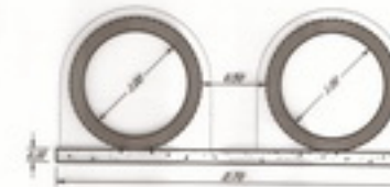
รูปตัดการวางท่อ คล.ล. ๒ และ ๓ ขนาดจริง 1 : 25
