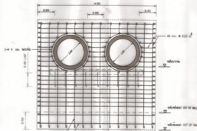
แบบขยายเหล็กเสริมคอนกรีตปากท่อด้านใน ขนาดจริง 1 : 25
