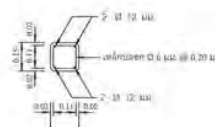
รูปตัด ข - ข
