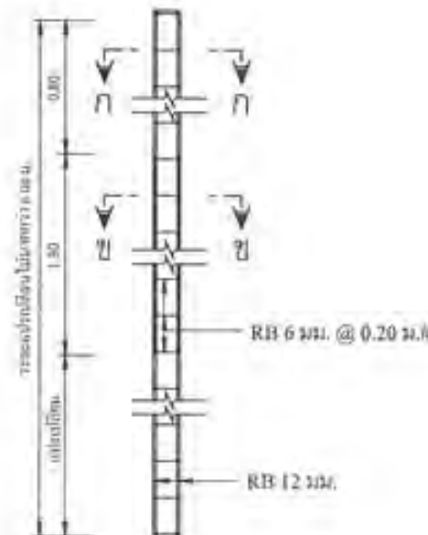
รายละเอียดเสาป้าย กสส.
