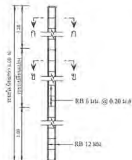
รายละเอียดค่างูปีน กสค. มกราคม 120
