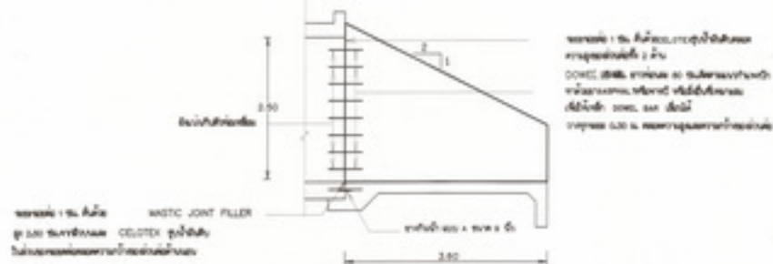
แบบแสดงรอยต่อระหว่างท่อน้ำเหลี่ยมกับปีกกำแพง
