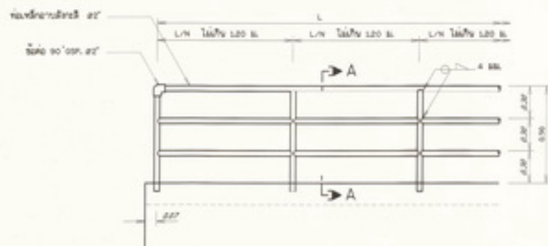
รูปขยายราวเหล็กกันดก มาตราส่วน 1:20
