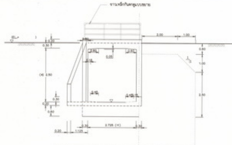
รูปตัด C - C
