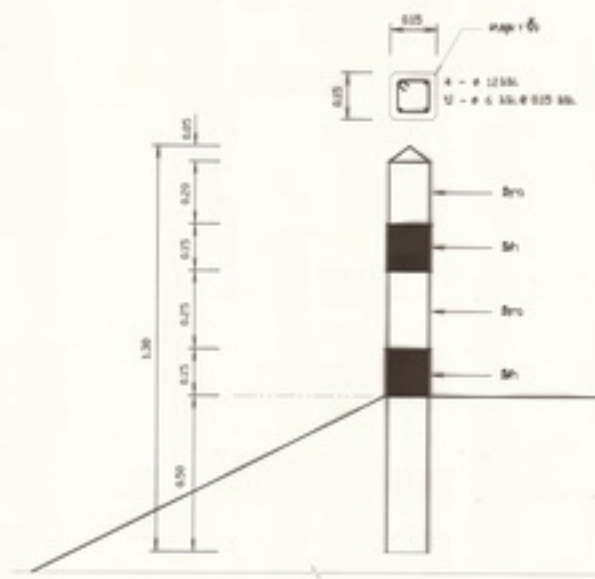
แบบขยายหักครึ่งคันดิน มาตราส่วน 1:10
