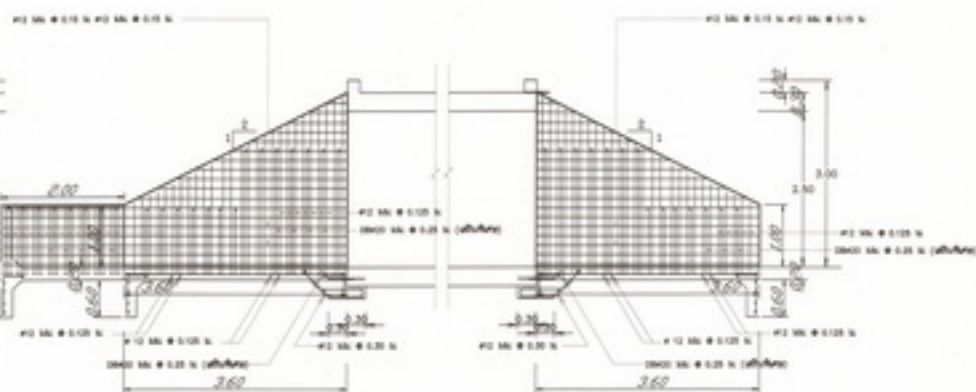
รูปตัดขยายการเสริมเหล็กแนว D - D
