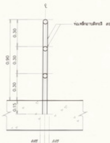
รูปตัด A - A มาตราส่วน 1:10
