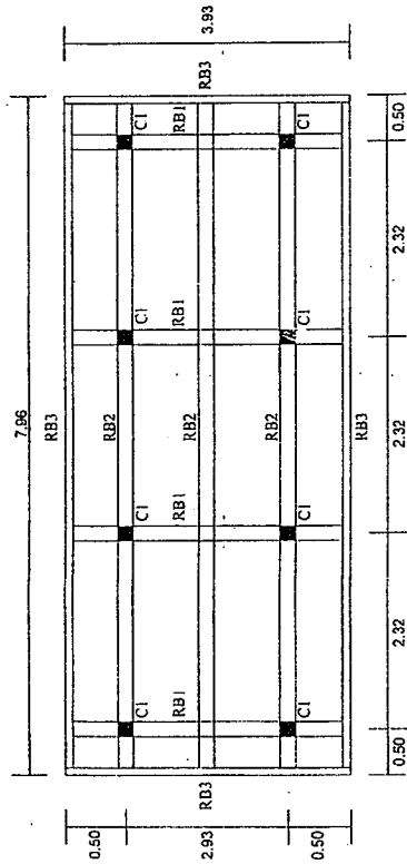
แปลนฐานรากและคานเหล็ก
