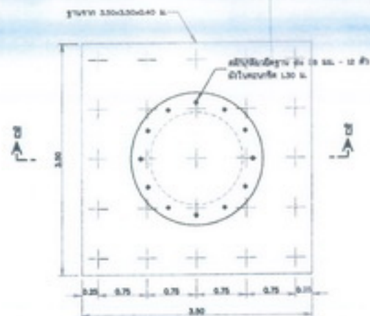
แปลน ฐานรากหอดังสูง (แบบเสาเข็ม) โมดูลสถาปัตย์
