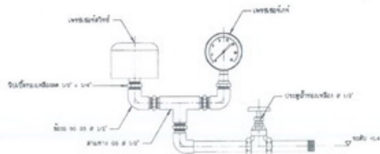
แบบขยายลิฟต์ควบคุมและเกจวัดความดัน ในสถานีฯ
