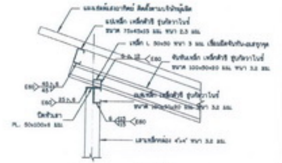
รูปขยาย การติดตั้งโครงหลังคา ไม่แสดงคานขวาง
