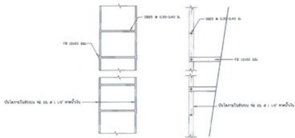
แบบขยายบันได ภายในห้องสูง ในสถานีฯ
