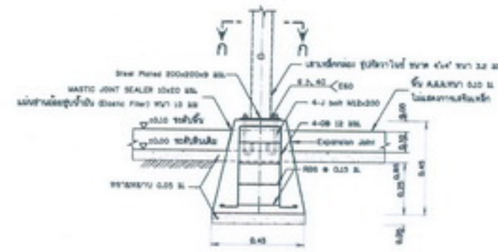
รูปขยายฐานรากโครงสร้างรับแผง F1 ขนาด 300x300 มม. พร้อมรูปหน้าตัด
