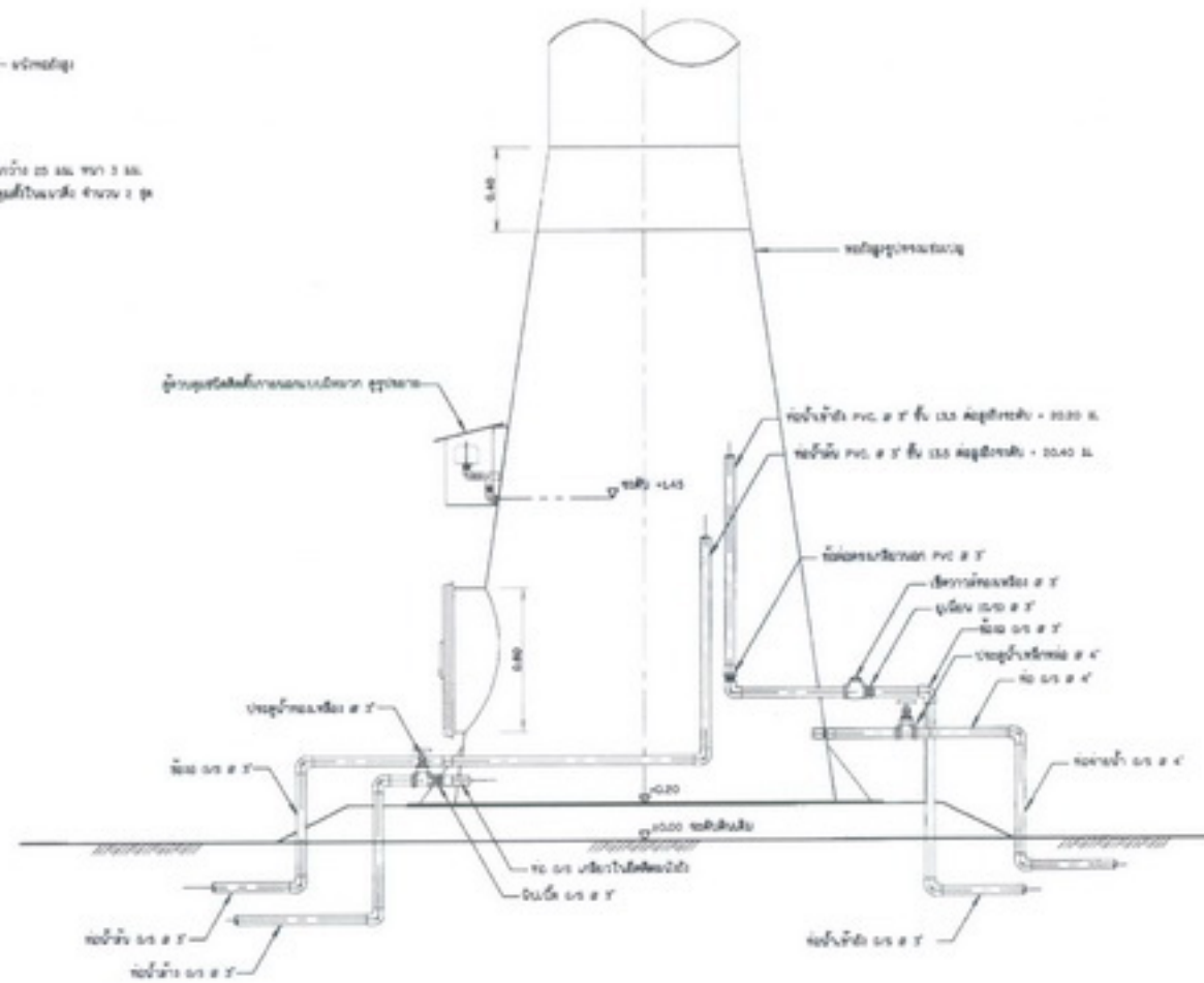
แบบแสดงการเดินท่อในห้องสูง ในสถานีฯ
