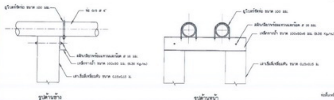
13. เสาคอมมิวนิตี้รับท่อ และแบบขยายอุปกรณ์รัดท่อ โมดูลมาตรฐาน
