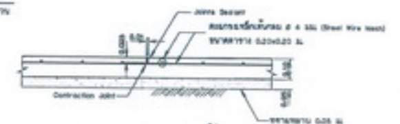
แบบขยายรอยต่อพื้น ไม่แสดงคานขวาง
