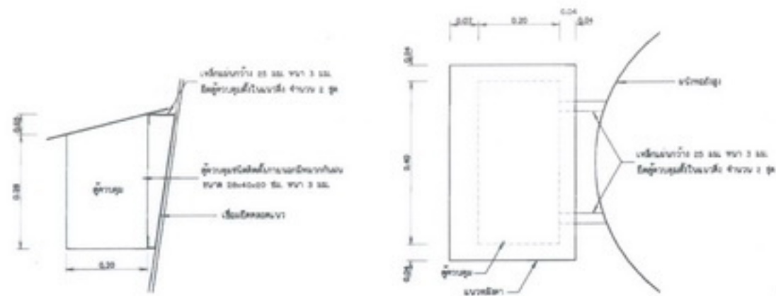
แบบขยายตู้ควบคุม ในสถานีฯ
