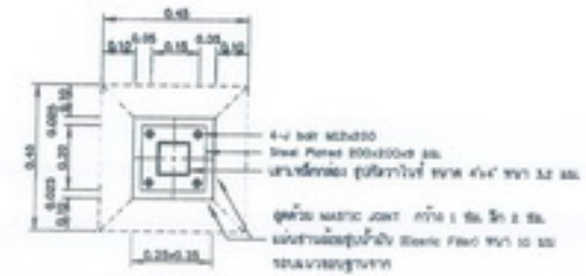
รูปตัด ก-ก ไม่แสดงคานขวาง
