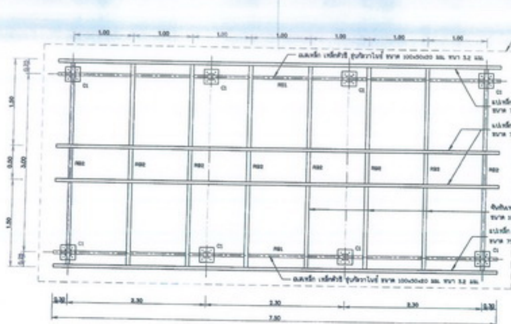
แปลนฐานรากและโครงหลังคา ไม่แสดงคานขวาง
