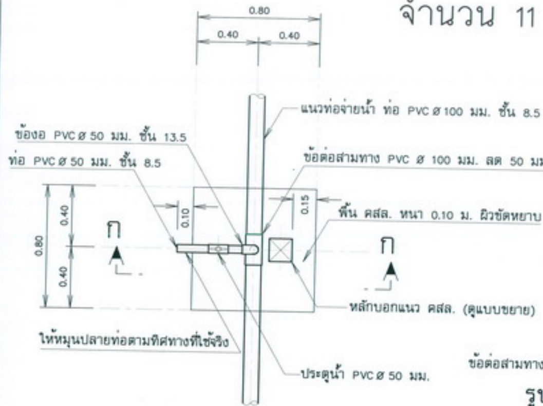
แบบแปลนอาคารจุดปล่อยน้ำ
