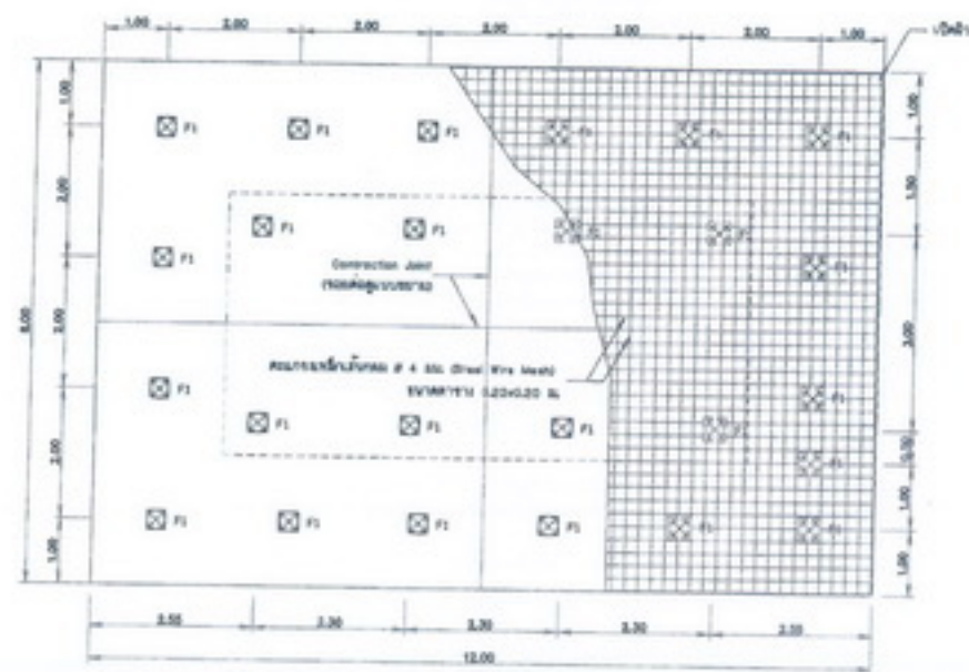
รูปขยายพื้นคอนกรีต ไม่แสดงคานขวาง
