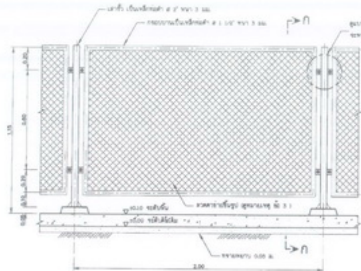
แบบขยายจั่วลดตาข่าย ไม่แสดงค่าส่วน
