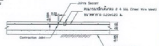
แบบขยายรอยต่อพื้น โมดูลมาตรฐาน
