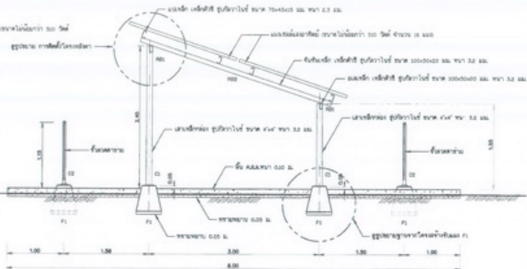
รูปด้านข้าง โมดูลมาตรฐาน
