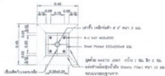
รูปตัด ข-ข ไม่แสดงค่าส่วน
