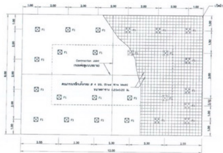
รูปขยายพื้นคอนกรีต โมดูลมาตรฐาน
