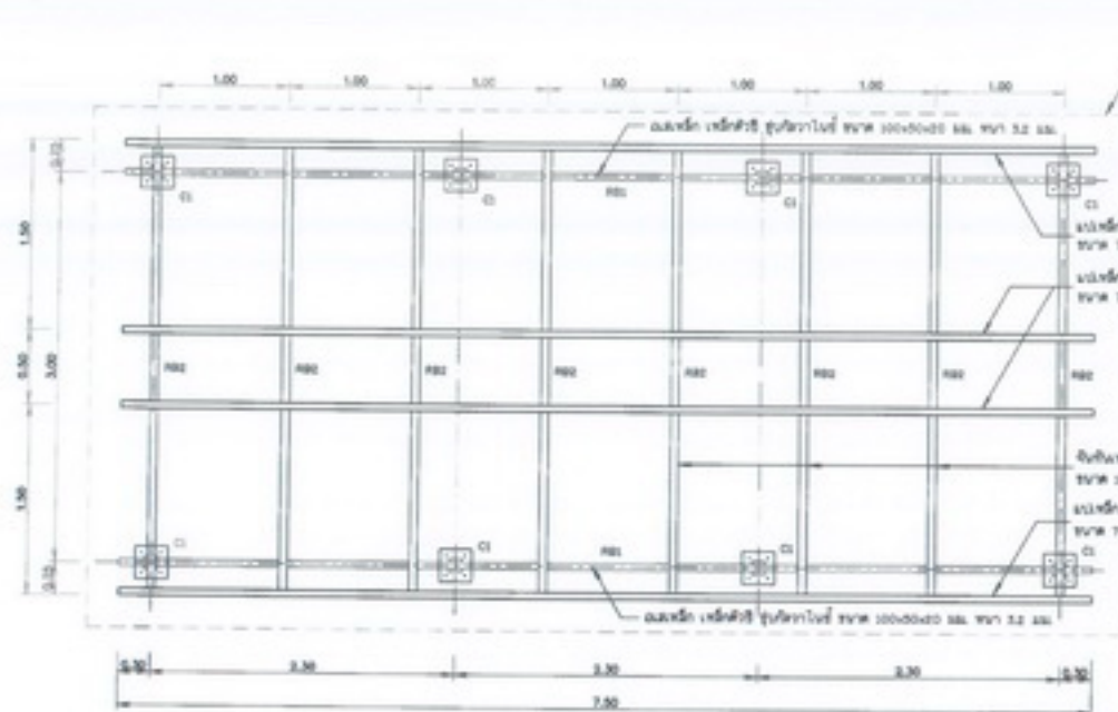
แปลนฐานรากและโครงหลังคา โมดูลมาตรฐาน
