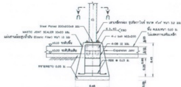
รูปขยายฐานรากจากโครงสร้างรับแรง F1 โมดูลมาตรฐาน
