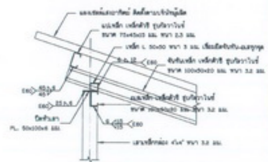
รูปขยาย การติดตั้งโครงหลังคา โมดูลมาตรฐาน
