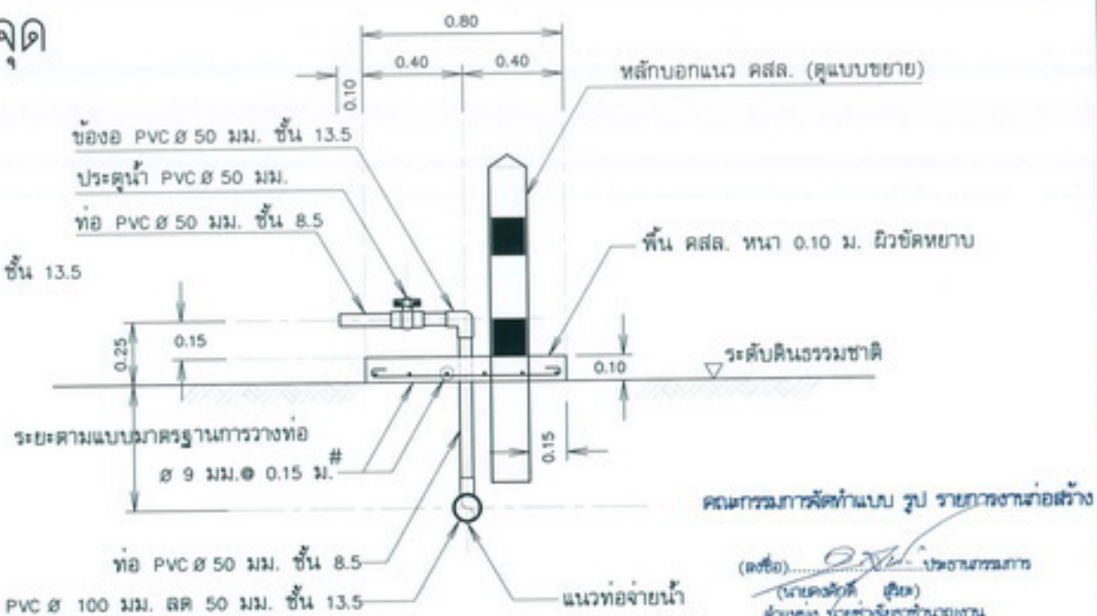
รูปตัด ก - ก แสดงการติดตั้งอาคารจุดปล่อยน้ำ
