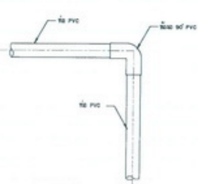
7. แบบการต่อข้ออ 90° PVC ไม่แสดงภาพส่วน
