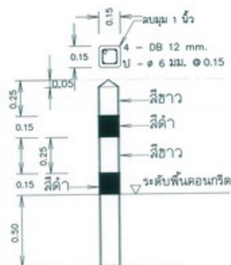
แบบขยายหลักบอกแนว
