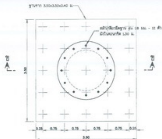
แปลน ฐานรากท่อถังสูง (แบบเสาเข็ม) ไม่แสดงทิศทาง
