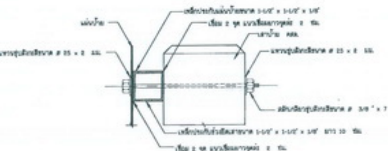
รูปตัดขยายการยึดแผ่นป้ายและเสา ไม่แสดงภาพตัว
