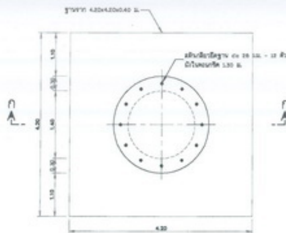
แปลน ฐานรากท่อถังสูง (แบบฐานแผ่) ไม่แสดงทิศทาง
