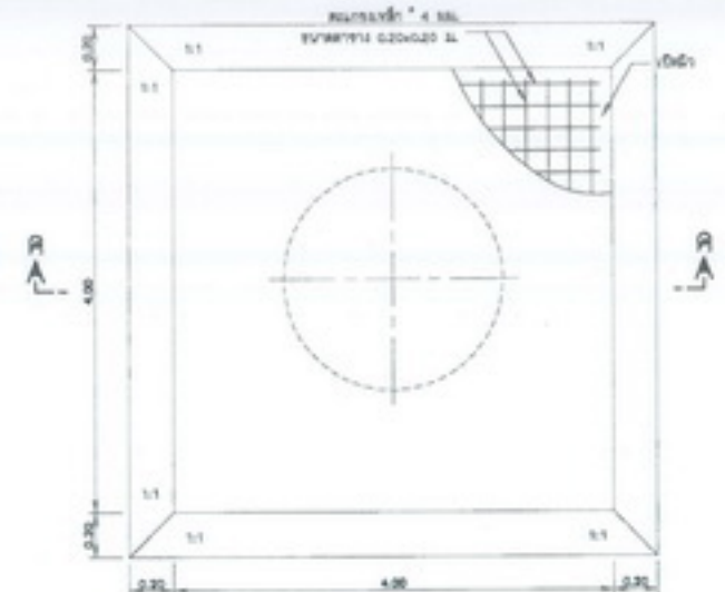
แปลน พื้นคอนกรีตเสริมเหล็ก ไม่แสดงทิศทาง
