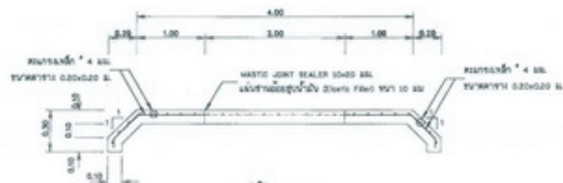
รูปตัด ค-ค ไม่แสดงทิศทาง
