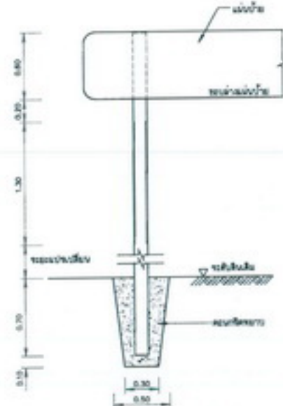
รายละเอียดการติดตั้งเสาป้าย ไม่แสดงภาพตัว
