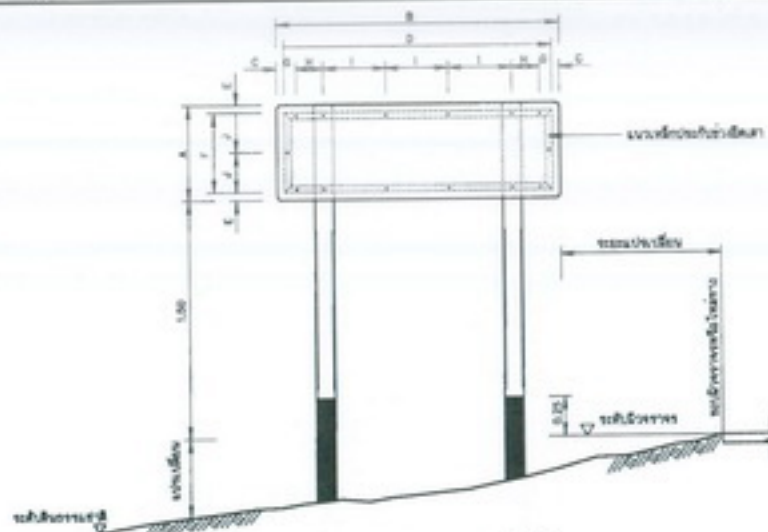
รูปแสดงการประกอบแผ่นป้าย ไม่แสดงภาพตัว
