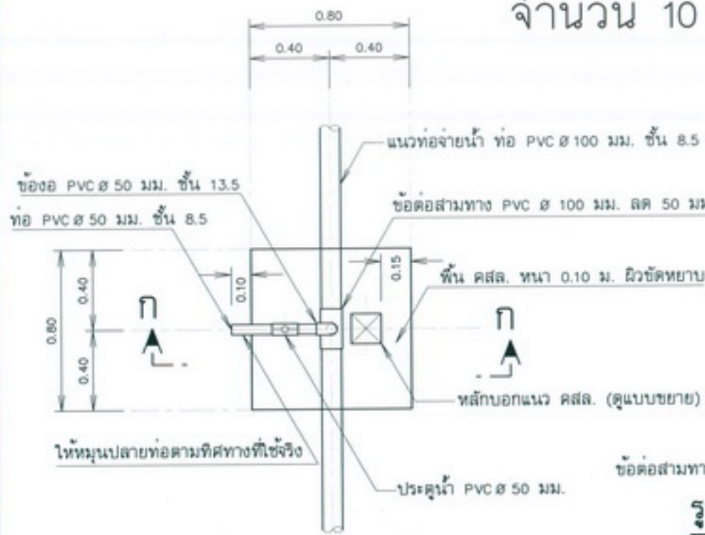
แปลนอาคารจุดปล่อยน้ำ
