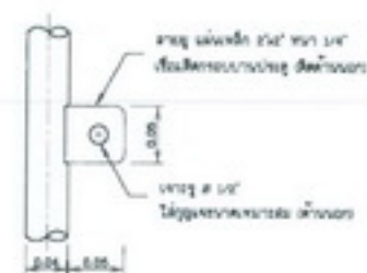
แบบขยายสาย ไม้มะยม
