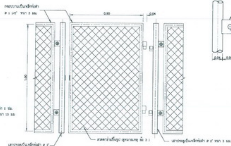
แบบขยายสาย ไม้มะยม
