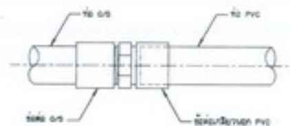
2. แบบการต่อท่อ G/S กับท่อ PVC ไม้มัดสายพาน
