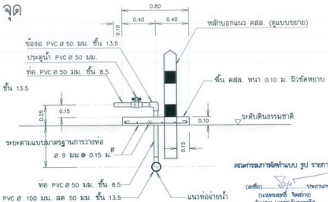
รูปตัด ก - ก แสดงการติดตั้งอาคารจุดปล่อยน้ำ
