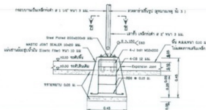
รูปขยายฐานจากโครงสร้างรับแผง F1 (ขนาด 300, 400 มม.) รูปถ่ายโดยผู้เขียน
