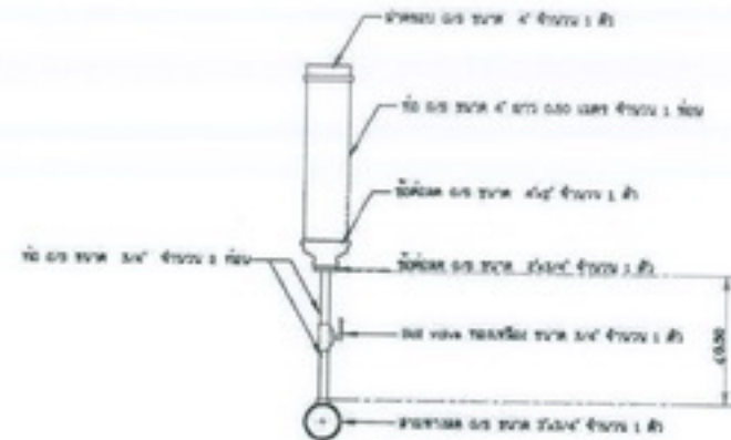
11. ช่องเดินน้ำ ไม่แสดงสายพาน
