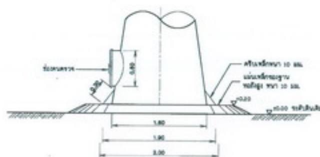
แบบขยายแมนโฮลล่างห่อถึงสูง
