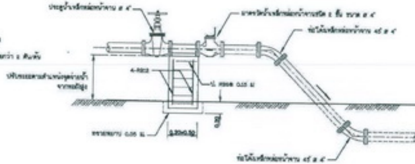
14. การติดตั้งมาตรวัดน้ำบนพื้นดิน ๘' 4" ไม่แสดงสายพาน
