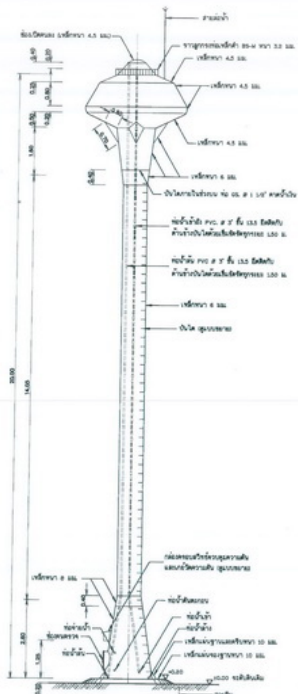
รูปด้านข้างหลอดสูง แบบตั้งเหลี่ยมรูปทรงแซมแปญ
