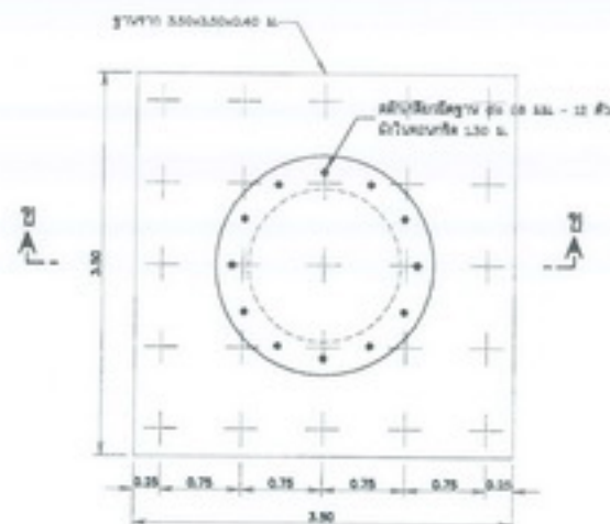
แปลน ฐานจากท่อถังสูง แบบเสาเข็ม ไม่แสดงค่าตัว
