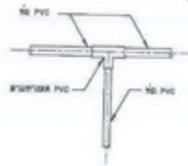
9. แบบการต่อสามทางลด PVC ไม่แสดงสายพาน
