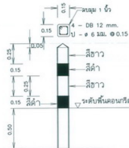
แบบขยายหลักบอกรูแนว
