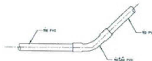
5. แบบการต่อข้อโค้ง 22 1/2, 45° PVC ไม้มัดสายพาน
