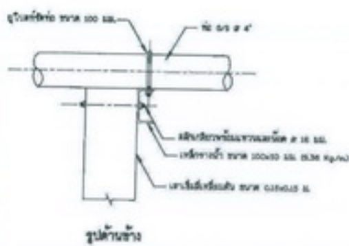
13. เสาคอมม่อนรับท่อชุด และแบบขยายอุปกรณ์วัดท่อ ไม่แสดงสายพาน
