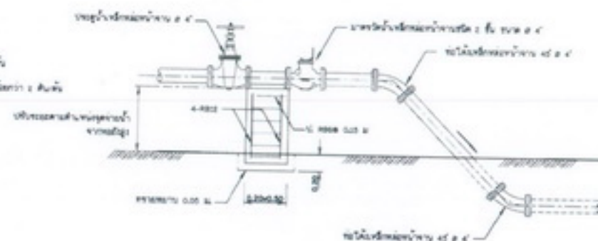
14. การติดตั้งมาตรวัดน้ำบนพื้นดิน ๑ 4" โมเดลมาตรฐาน
