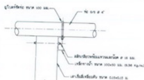
รูปด้านข้าง
