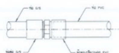
2. แบบการต่อท่อ G/S กับท่อ PVC ในเขตเทศบาล
