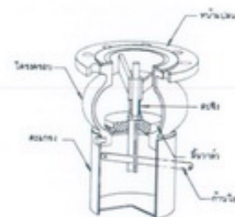
ชุดวาล์ว แบบกันโยก โมเดลมาตรฐาน
