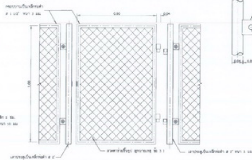
แบบขยายสายยู ในเล่มประกอบ
